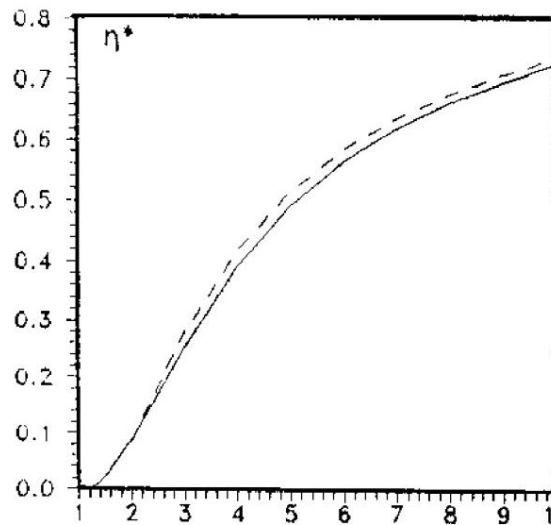
Figure 1.5 : Rendement * du ressaut classique en fonction du nombre de Froude. (—) Courbe tracée selon la relation (1.21). (---) Courbe tracée selon la relation (1.22).
