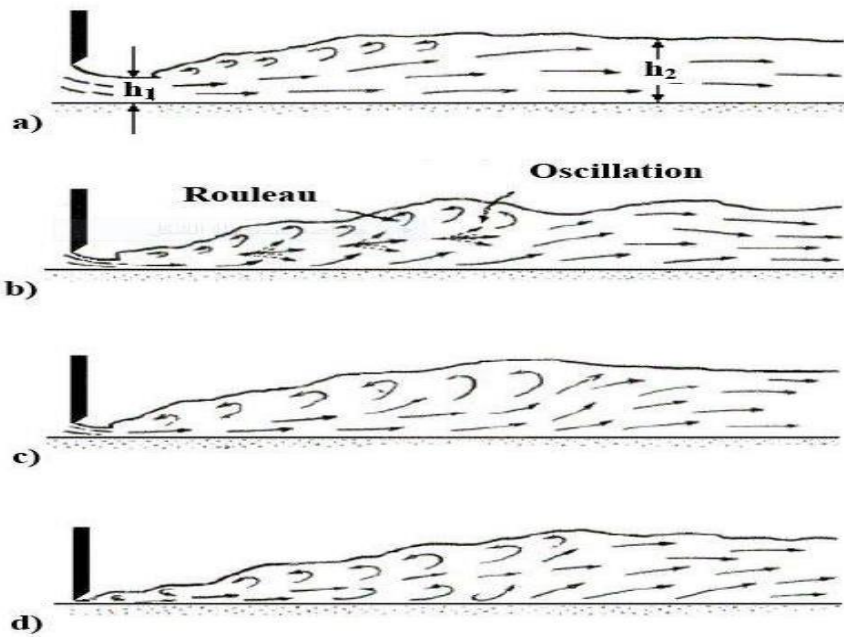
Figure 1.1 : Forme du ressaut classique selon la classification de Bradley et Peterka (1957). a) pré-ressaut, b) ressaut de transition, c) ressaut stable et d) ressaut agité.
