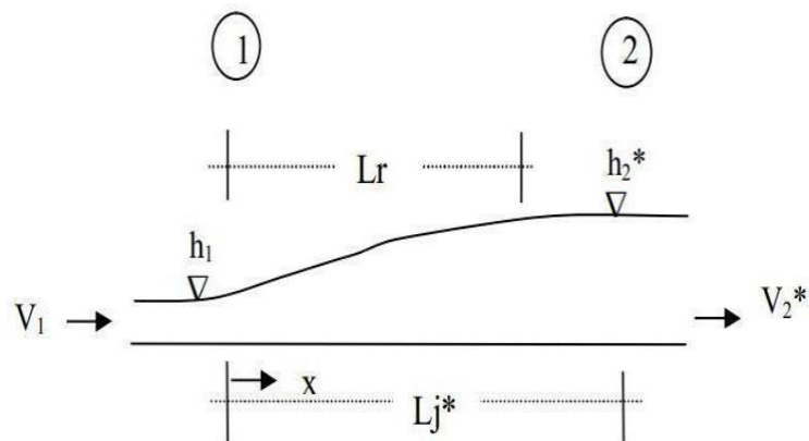
Figure 1.2 : Resson hydraulique classique.
