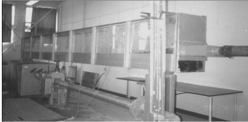
Photo 2.3: Dispositif expérimental ayant servi à l'étude du ressaut contrôlé par un seuil dans un canal rectangulaire.
