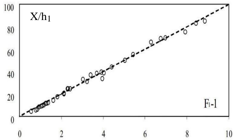
Figure 2.12 : Variation expérimentale de la position relative X/h_1 du seuil à paroi mince en fonction de (F_1 - 1) lors du contrôle du ressaut dans un canal rectangulaire ( X \cong L_j ). ( - - - ) courbe tracée selon la relation (2.8).
