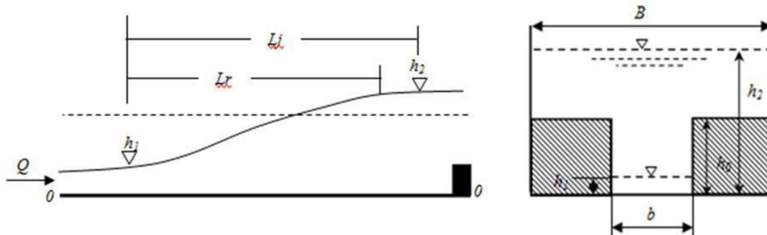
Figure II.1 : Schéma simplifié d'un ressaut hydraulique contrôlé par seuil évoluant dans un canal rectangulaire composé.
