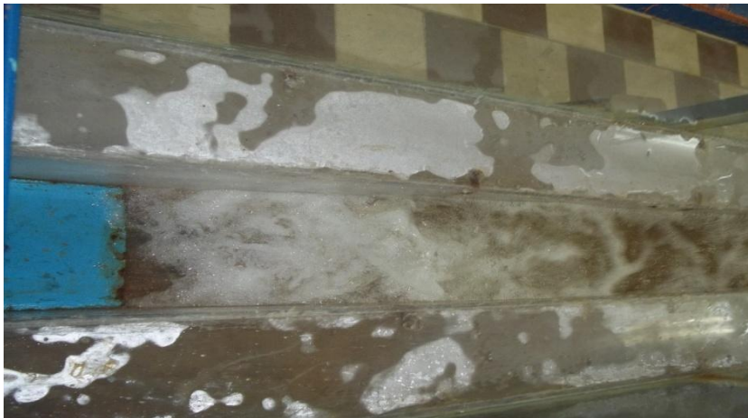
Photo II.1 : Photographie d'un ressaut hydraulique contrôlé par seuil mince F_1 = 5,58 ; s = 6 cm; h_2 = 15,8 cm ; h_1 = 2,5 cm
