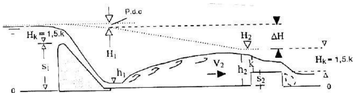
Figure II.16 : Ressaut contrôlé par un seuil à paroi épaisse à l'aval d'un déversoir standard. P.d.c : pertes de charge sur le parement aval du déversoir.
