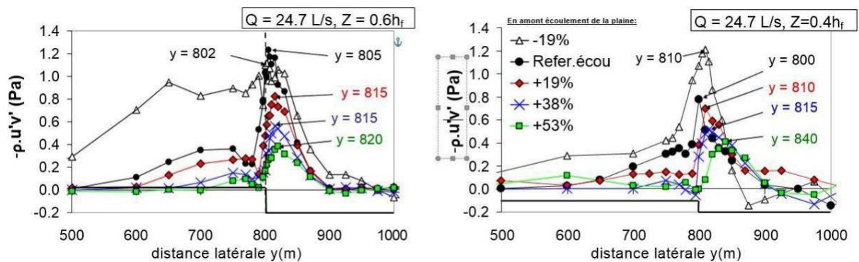
Figure 3.9 : Position des pics de la contrainte de Reynolds xy pour le débit Q = 24,7 L/s, à deux altitudes différentes: Z = 0.6 h_f et 0.4 h_f
