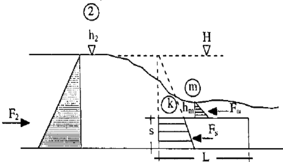
Figure 2.13 : Écoulement franchissant un seuil épais continu de hauteur s et de longueur L . Les parties hachurées correspondent à la répartition supposée hydrostatique des pressions.
