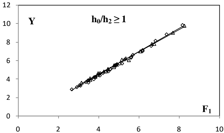
Figure II.4 : variation du rapport Y des hauteurs conjuguées du ressaut hydraulique en fonction du nombre de Froude F_1 , pour les deux configurations. Pour h_0/h_2 \geq 1 . ( \diamond ) seuil mince, ( \Delta ) seuil épais.
