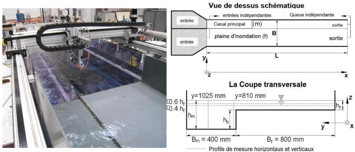
Figure 3.6 : Canal de canal composé à LMFA (le schéma n'est pas à l'échelle)
