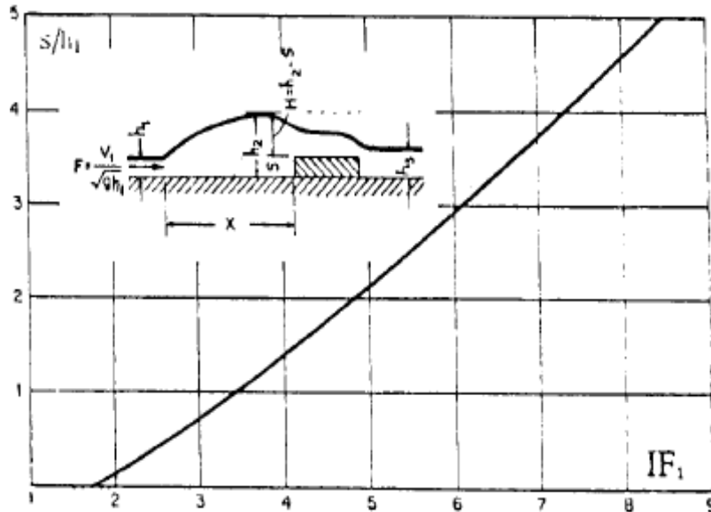
Figure II.14 : Variation expérimentale du nombre de Froude IF_1 en fonction de la hauteur relative s/h_1 du seuil à paroi épaisse, selon Forster et Skrinde (1950). Courbe tracée selon la relation (2.10).
