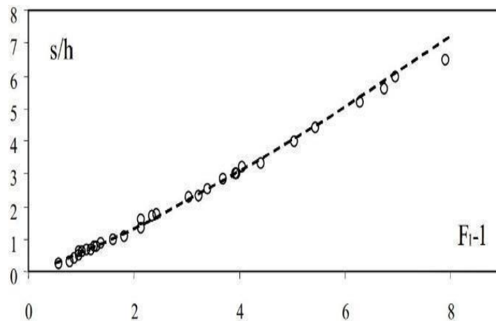
Figure 2.10 : Variation expérimentale de la hauteur relative s/h_1 du seuil à paroi mince en fonction du nombre de Froude F_1 de l'écoulement incident ( X \cong L_j ). (- - -) courbe tracée selon la relation (7).
