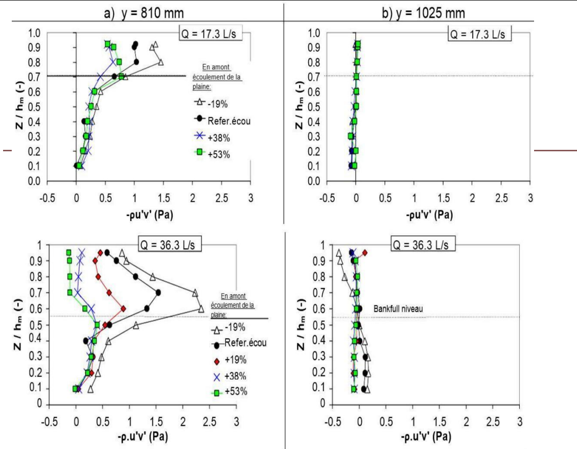
Figure 3.12 : Profils verticaux de la contrainte de Reynolds \tau_{xy} à deux positions latérales dans le canal principal: a) y = 810 mm et b) y = 1025 mm .Station aval x = 4,5 m
