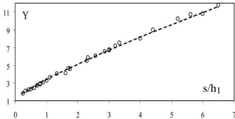
Figure 2.9 : Variation expérimentale du rapport Y des hauteurs conjuguées du ressaut en fonction de la hauteur relative s/h_1 du seuil à paroi mince ( X \cong L_j ) (- - -) courbe tracée selon la relation (6).
