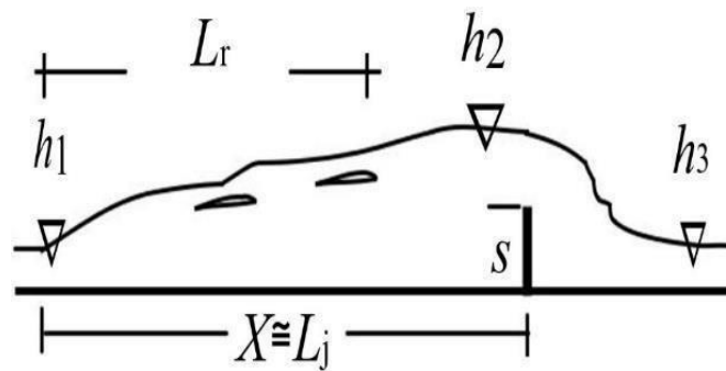
Figure 2.7 : Contrôle du ressaut par un seuil à paroi mince pour X \approx L_j
