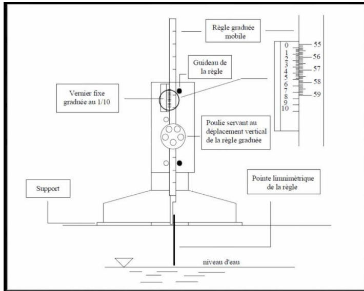
Figure I.3 : Mesure de la profondeur d'eau par pointe limnimétrique
