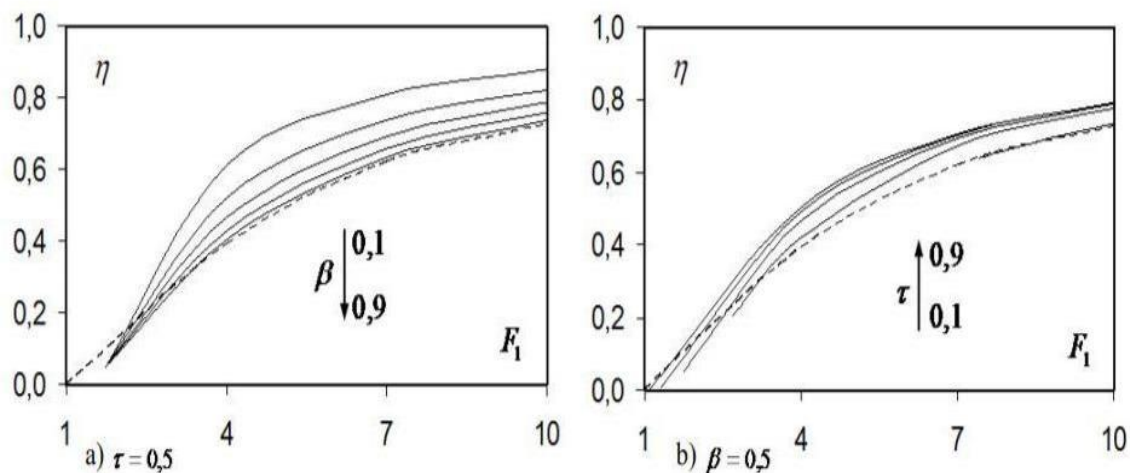
Figure 3.4 : Variation de \eta en fonction de F_1 . (- - -) : \beta = 1 . \eta est calculé par l'équation (3).
