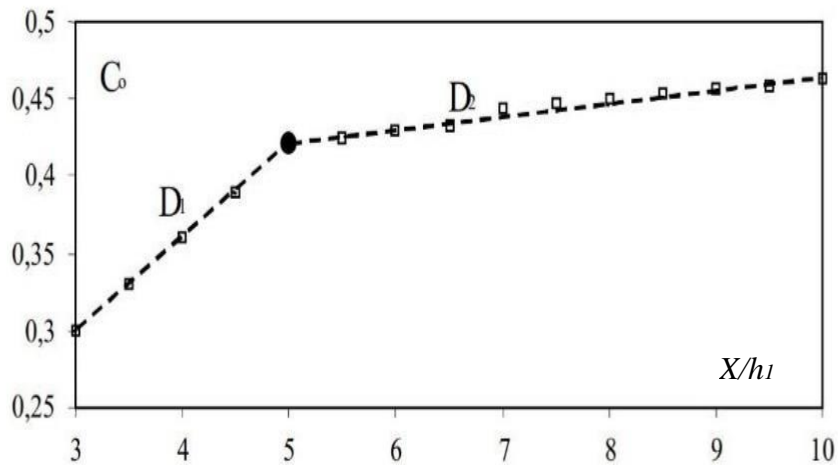
Figure 2.5 : Variation expérimentale de Coen fonction de la position relative X/h_1 du seuil à paroi mince.
