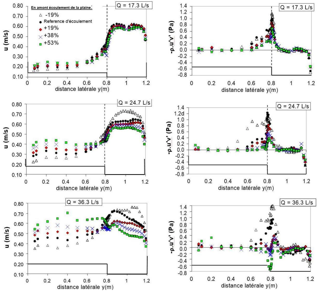
Figure 3.8 : Vitesse moyennes u et Reynolds de contrainte xy vs distance latérale. Profil horizontal à l'élévation Z = 0.6 h_f . Station aval x = 4,5 m
