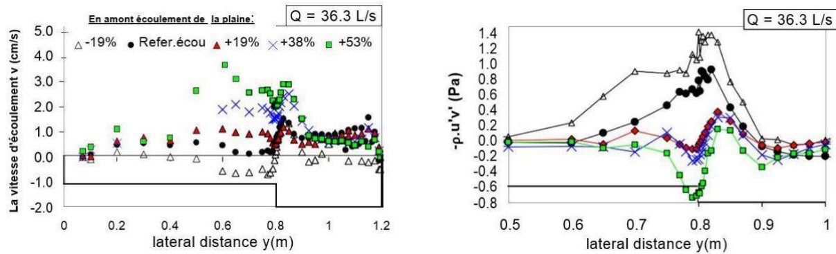
Figure 3.10 : Vitesse envergure v et contrainte de Reynolds \tau_{xy} à l'élévation 0.6h_f pour le débit Q = 36,3 \text{ L/s} et station aval x = 4,5 \text{ m}
