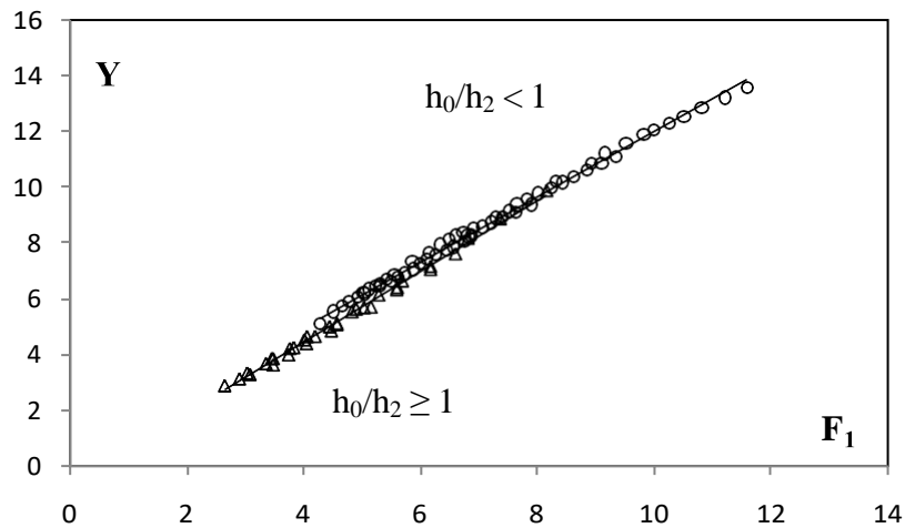
Figure. II.2. Variation du rapport Y des hauteurs conjuguées en fonction du nombre de Froude F_1 pour les deux lits du canal, (o) points de mesures expérimentales en lit majeur; ( \Delta ) points de mesures expérimentales en lit mineur. (—) Courbes d'ajustement.
