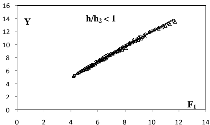
Figure II.5 : variation du rapport Y des hauteurs conjuguées du ressaut hydraulique en fonction du nombre de Froude F_1 , pour les deux configurations. Pour h_0/h_2 < 1 . ( \diamond ) seuil mince, ( \Delta ) seuil épais.
