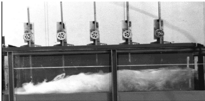
Photo 2.8 : Ressaut contrôlé par un seuil à paroi mince dans un canal rectangulaire F_1 = 7,74 , h_1 = 2,5 cm, s = 14 cm et X = 184 cm.
