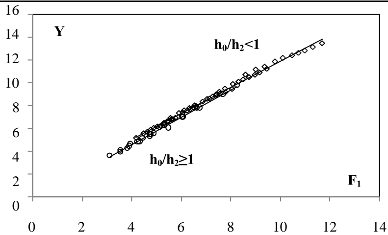
Figure. II.3. Variation du rapport Y des hauteurs conjuguées en fonction du nombre de Froude F_1 pour les deux cas du canal, (o) points expérimentaux (—) Courbes d'ajustement.
