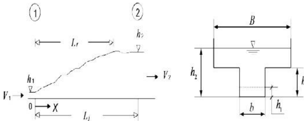
Figure I.1 : Schéma de définition du ressaut contrôlé par seuil continu à paroi mince
