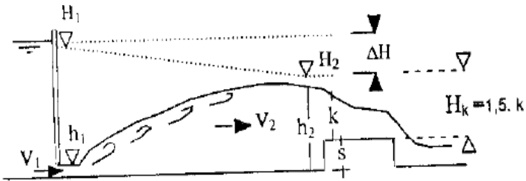
Figure II.15 : Ressaut contrôlé par un seuil à paroi épaisse à l'aval d'une vanne de fond, selon ACHOUR (1998).
