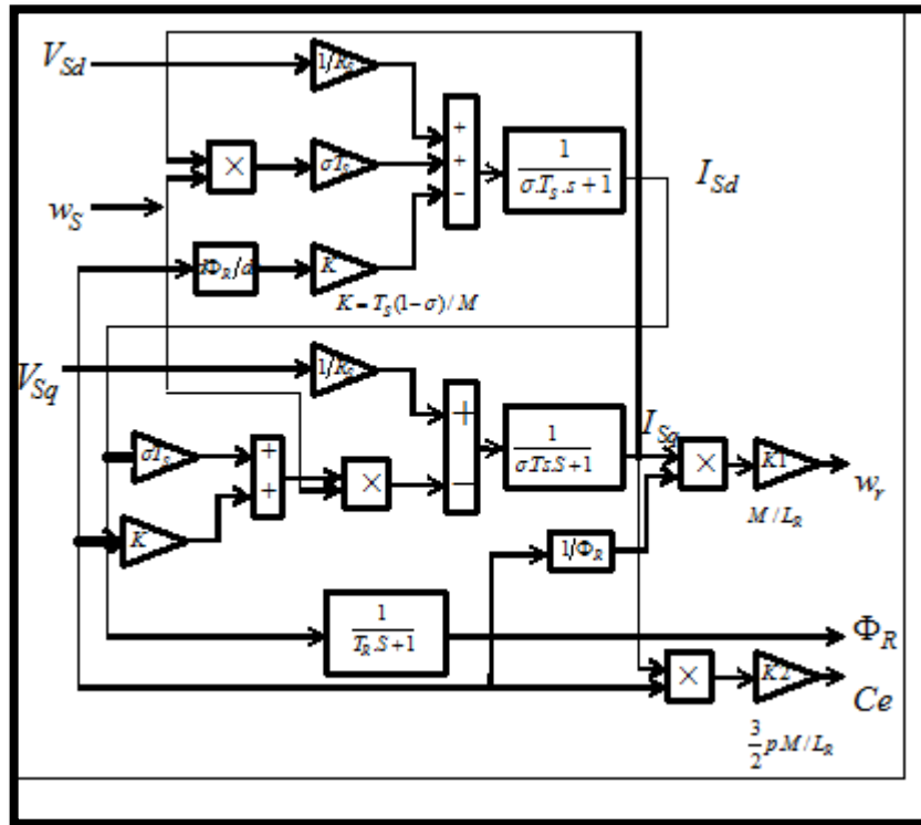
Fig. II- 2 : structure de la commande par orientation du flux rotorique
