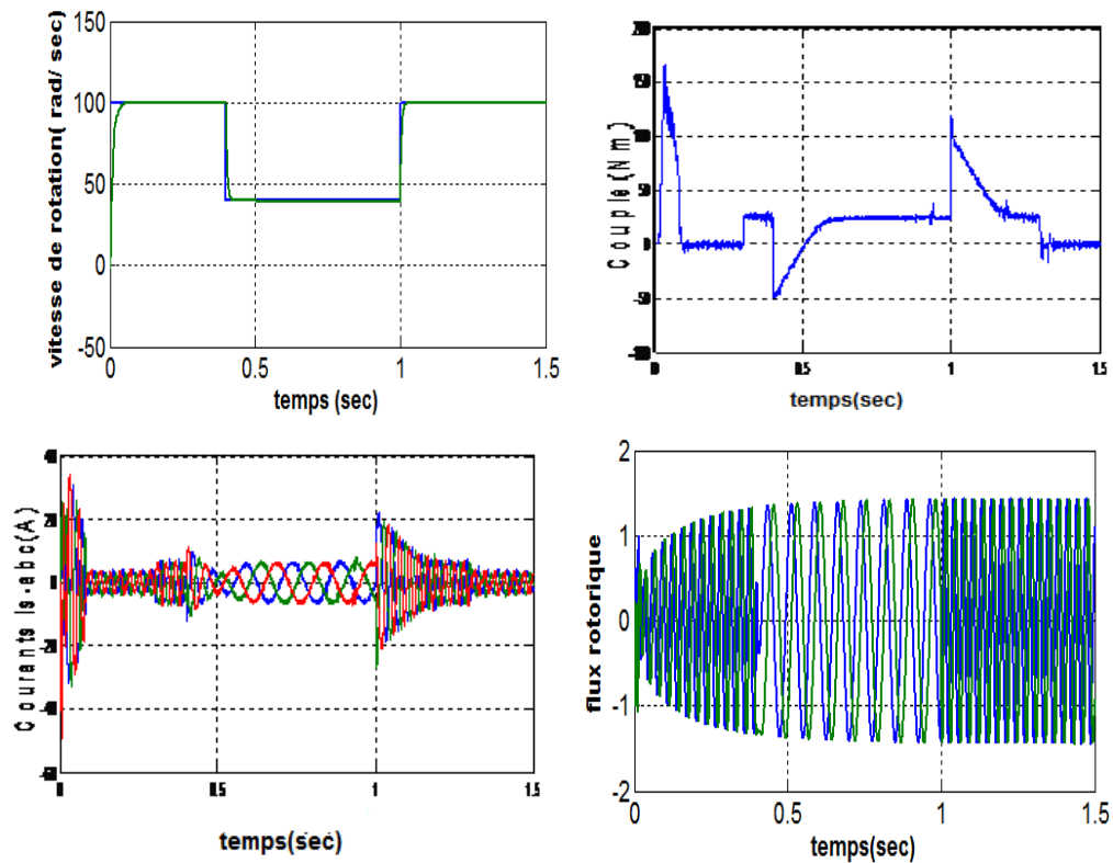
Fig. III- 12 :Test de variation de vitesse avec une application d'un couple de charge
