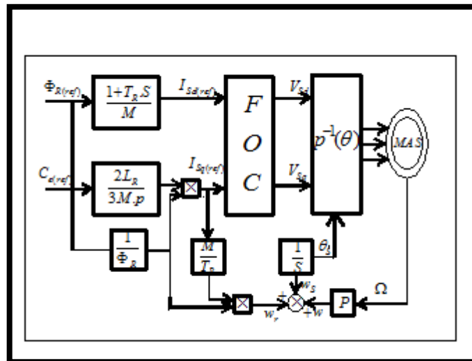
Fig. II- 4 : commande par orientation du flux avec découplage entrée sortie
