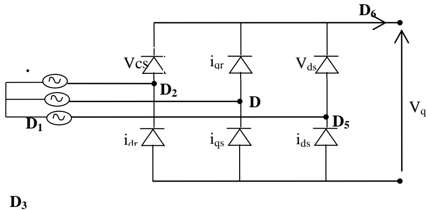
Fig. I- 6 : Représentation de la redresseuse triphasée double alternance.
