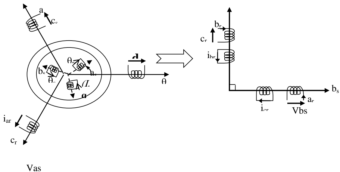
Fig. I- 4 : Modélisation de la machine asynchrone dans le repère de Park
