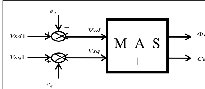
Fig. II- 3 : Reconstitution des tensions V_{sd} et V_{sq}
