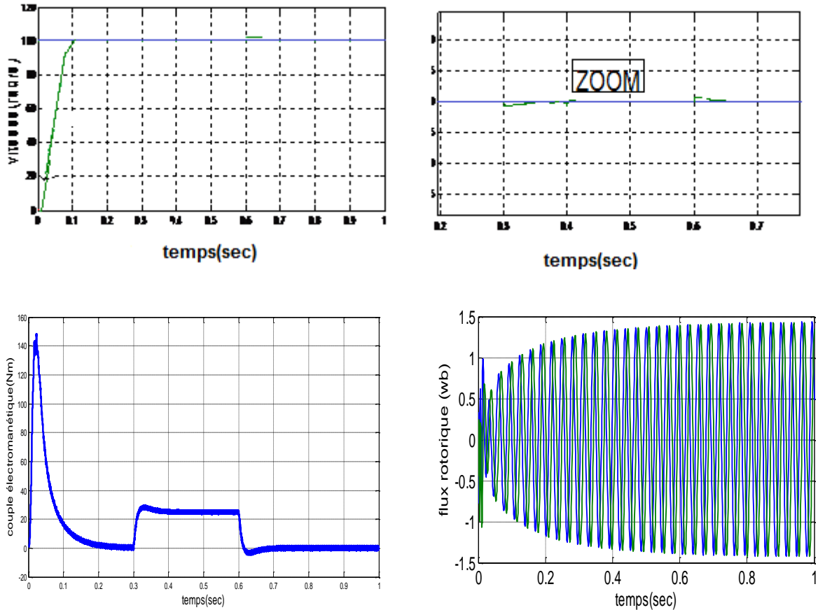
Fig. III- 10:Test un démarrage avec variation de la charge.
