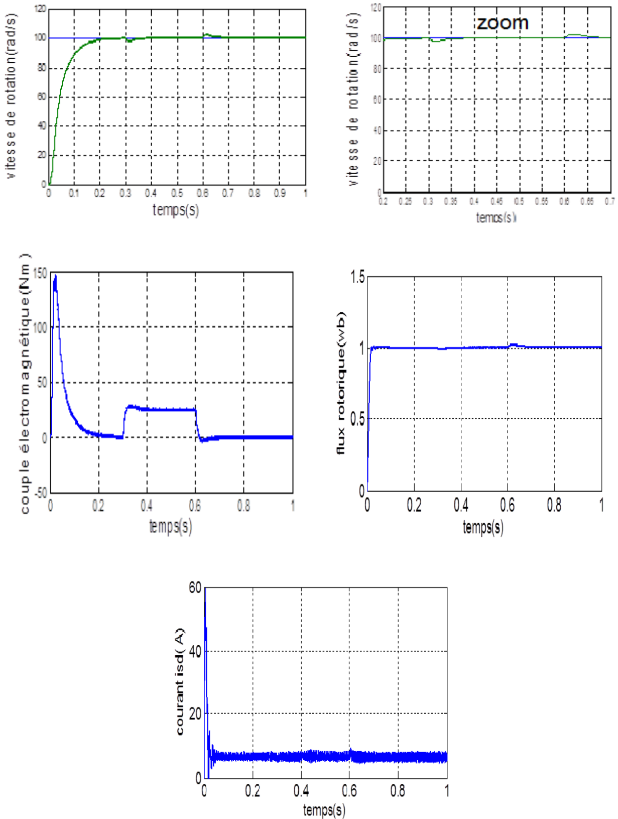
Fig. II- 14 : Simulation avec variation de la charge
