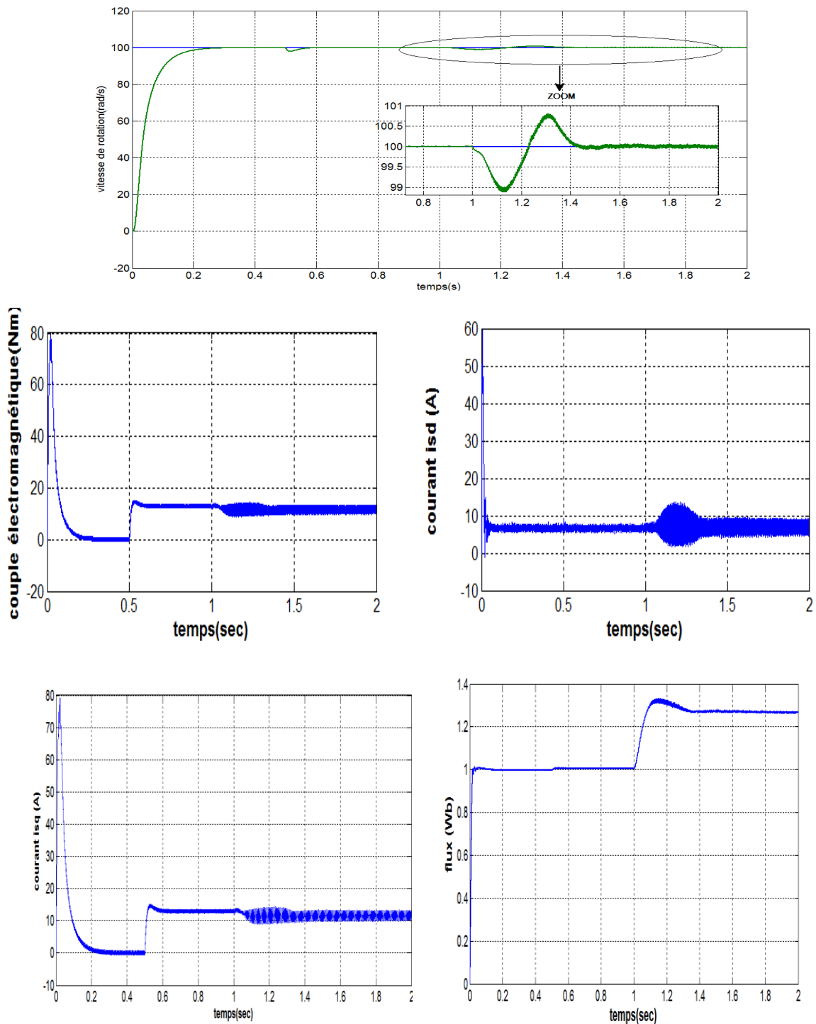
Fig.(II.16) Test de robustesse avec la variation de la résistance rotorique
