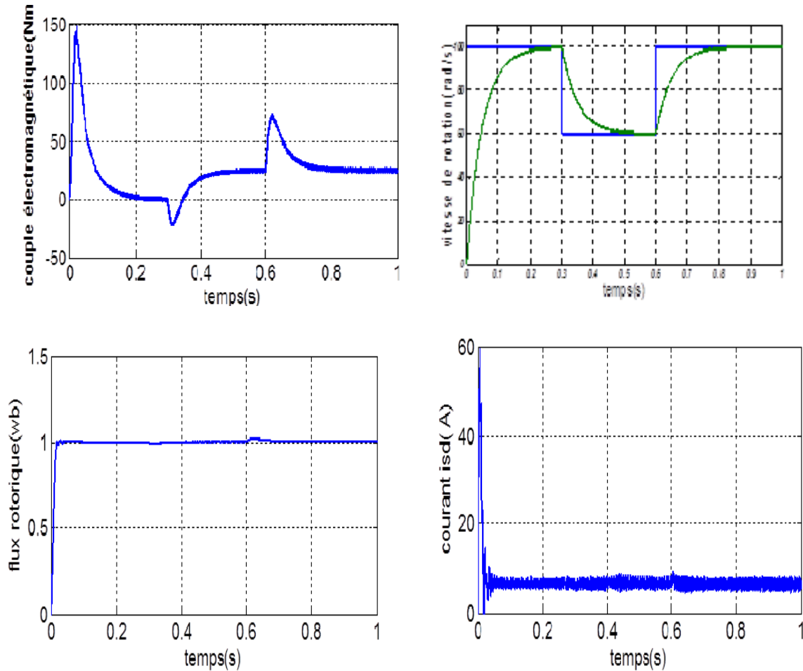
Fig. II- 12 Simulation avec variation de vitesse
