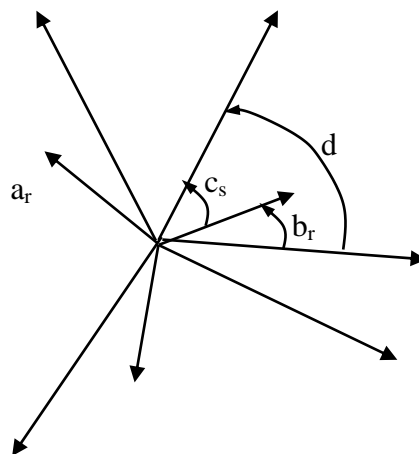
Fig. I-3 : Représentation des axes de la machine.
