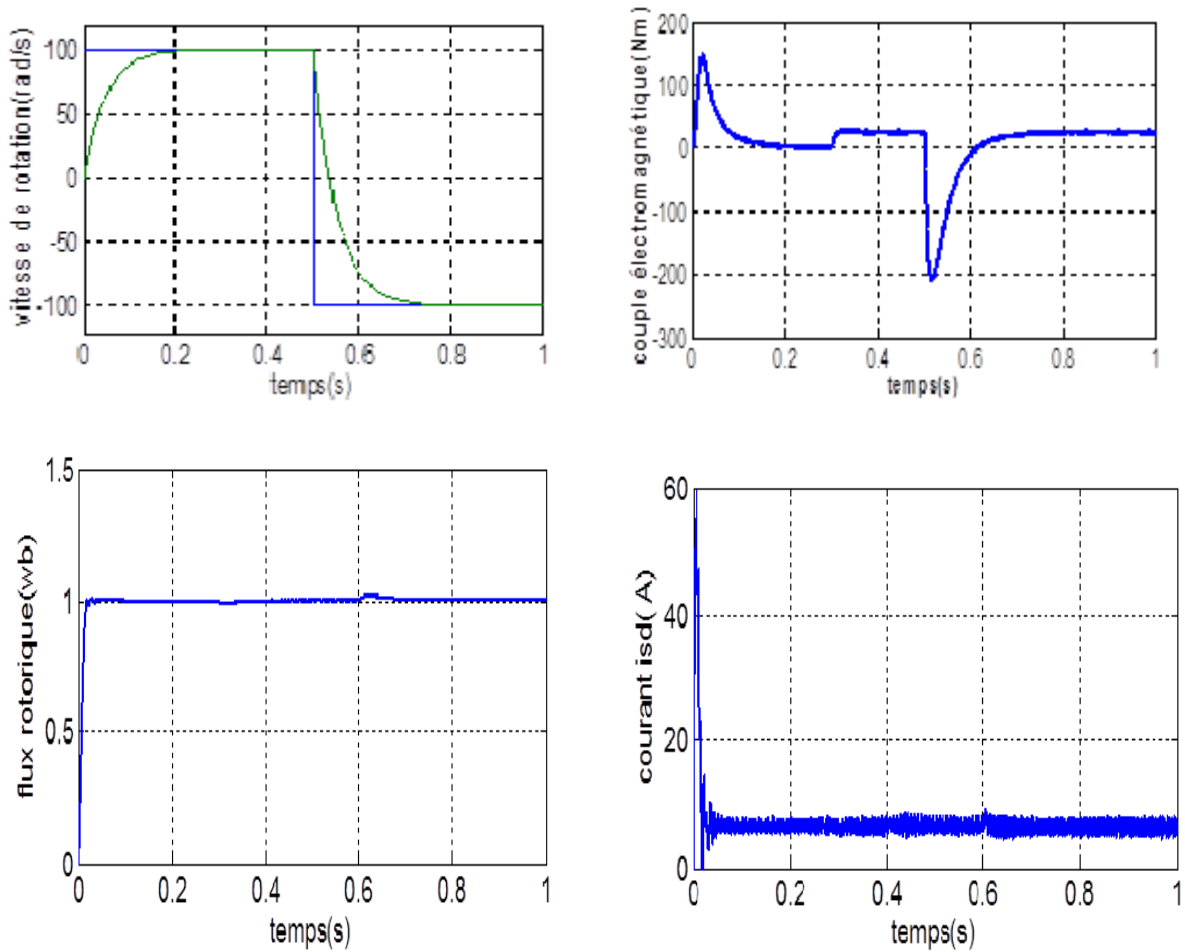
Fig. II- 13 : Simulations avec l'inversion de vitesse
