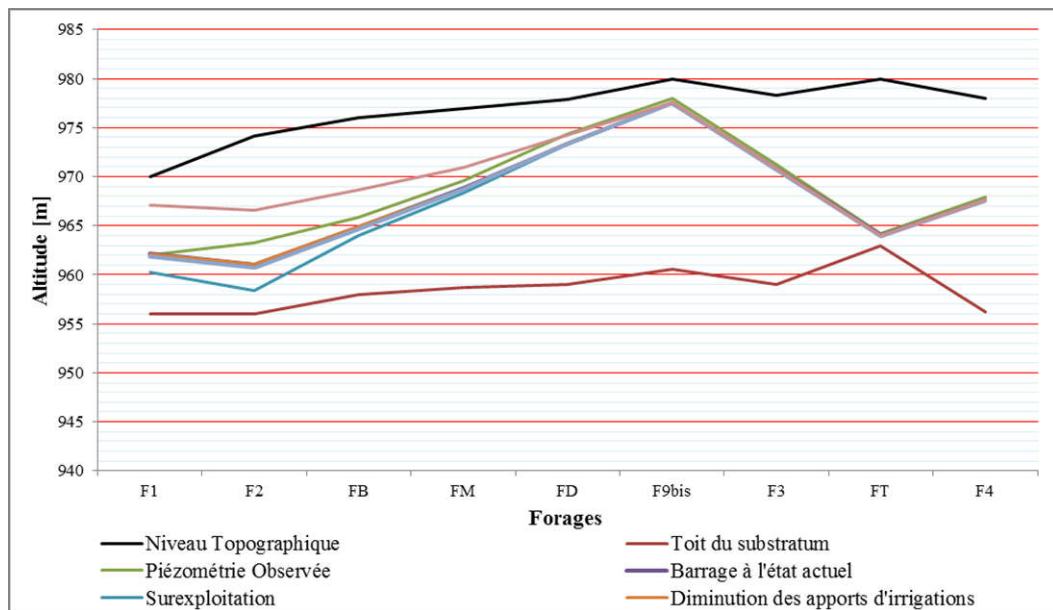
Fig.18. Évolution piézométrique simulée au niveau des forages avec barrage inféroflux
