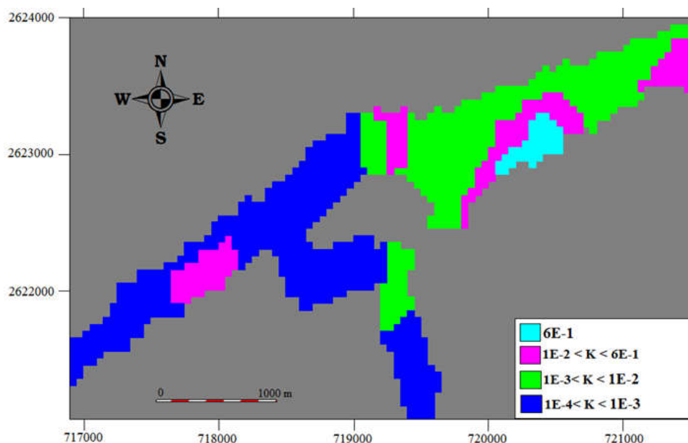
Fig.13.: Carte de la perméabilité (m/s) adoptée pour le calage en régime permanent.
