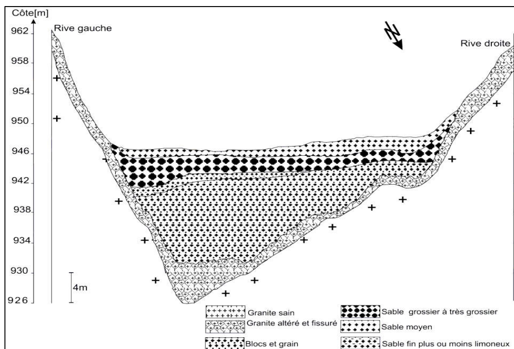
Fig. 5. Coupe hydrogéologique d'oued In Amguel, réalisé sur l'axe du barrage inféroflux.
