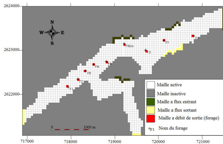
Fig. 10. Maillage et conditions aux limites du domaine à modéliser
