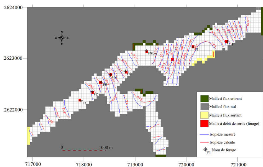
Fig. 11. Superposition et comparaison entre la piézométrie calculée et mesurée en régime permanent.
