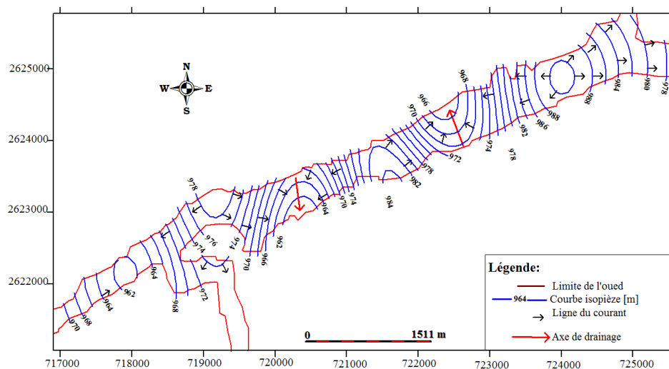
Fig. 7. Carte piézométrique de la nappe de l'inféoflux d'oued In Amguel (Février, 1986)
