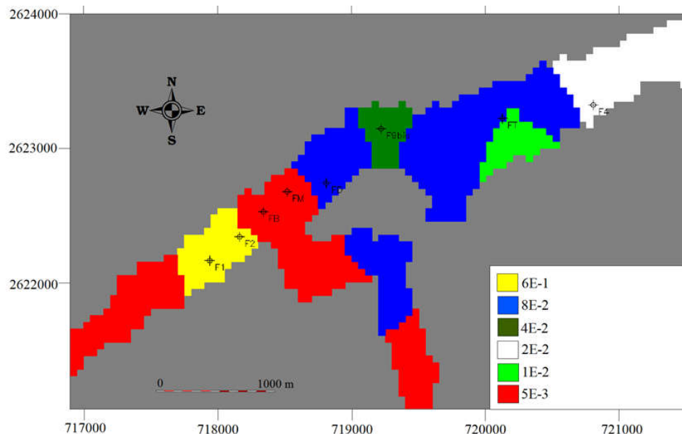
Fig. 16. Distribution des valeurs du coefficient d'emmagasinement adoptée pour le calage en régime transitoire.
