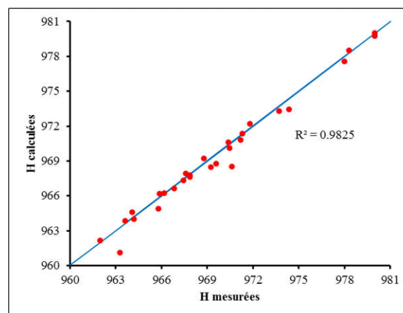
Fig. 14. Comparaison entre les potentiels mesurés et calculés après calage du modèle
