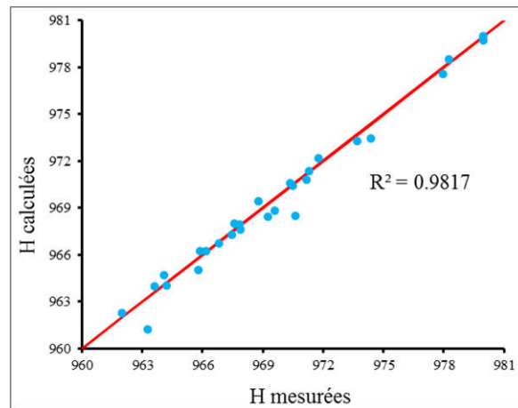
Fig .12. Comparaison entre les potentiels mesurés et calculés après calage du modèle en régime permanent.
