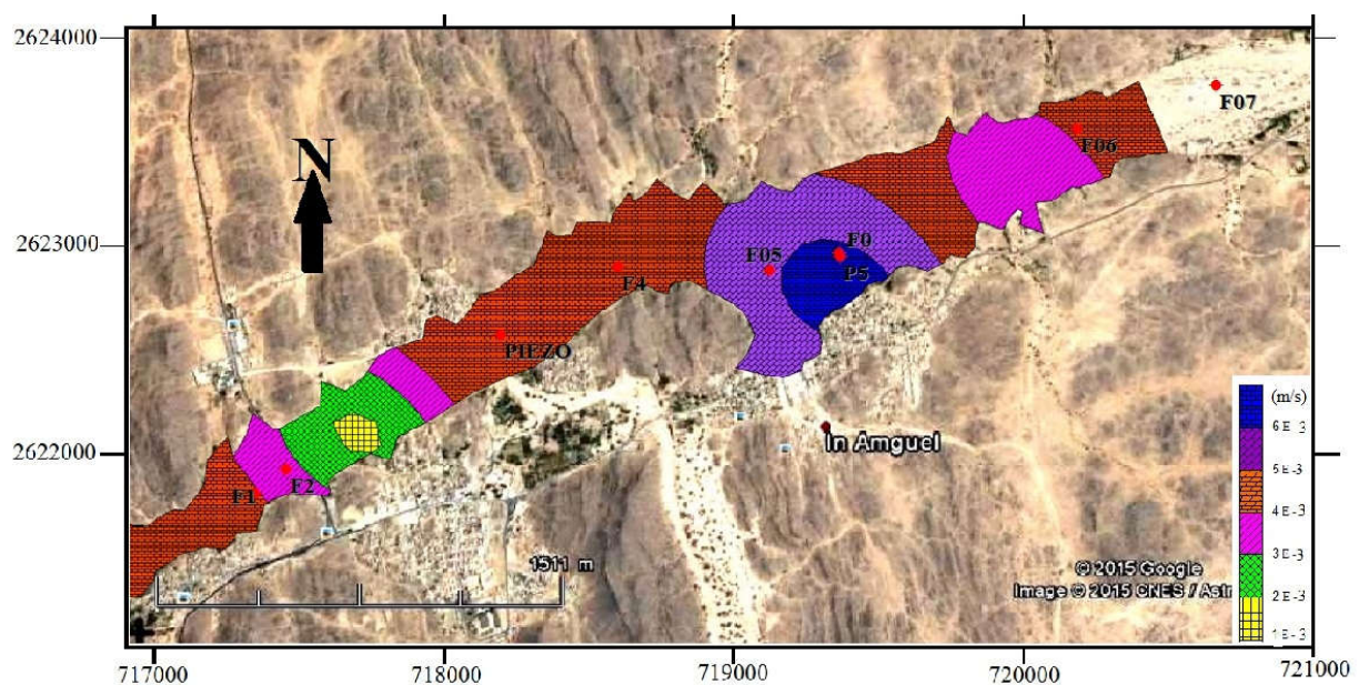
Fig. 9. Carte de perméabilité de l'aquifère inféroflux d'oued In Amguel (m/s)
