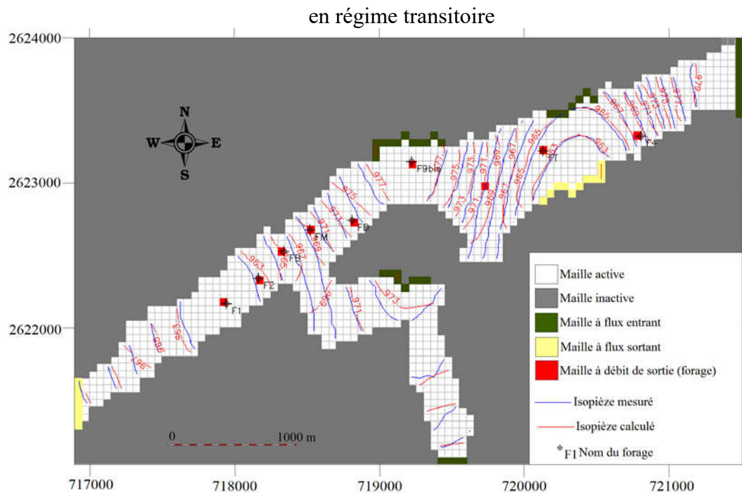
Fig. 15. Superposition des hydro-isohypses observées (février 1986) et calculées en régime transitoire.
