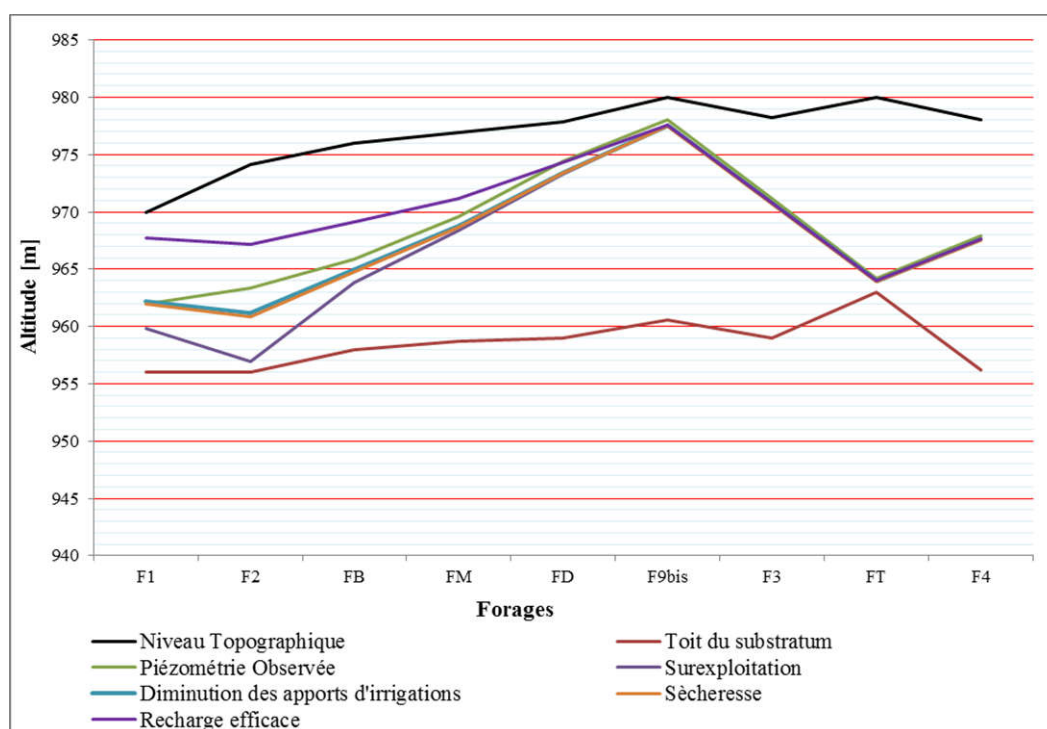
Fig.17. Évolution piézométrique simulée au niveau des forages sans barrage inféroflux
