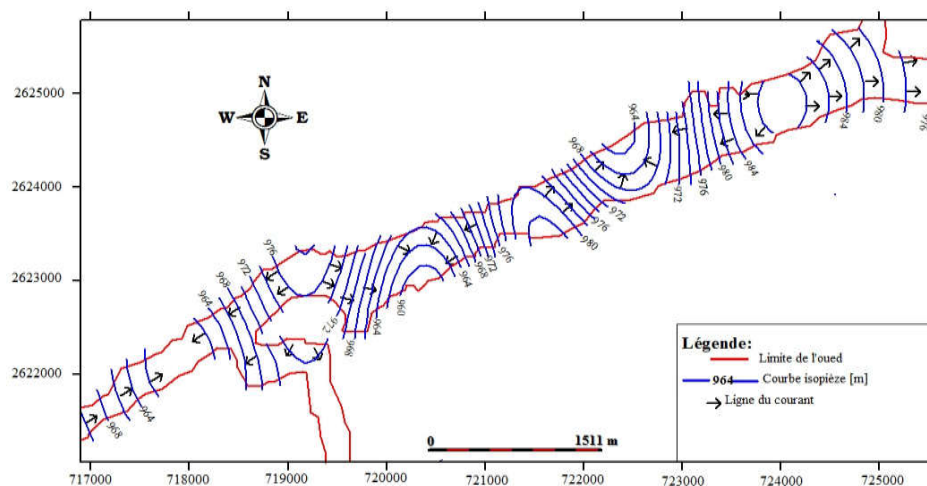
Fig. 7. Carte piézométrique de la nappe de l'inféoflux d'oued In Amguel (Février, 1986)
