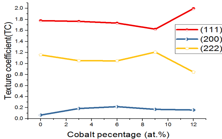
الشكل (8.III): قيم معامل النسيج لجميع قمم الأغشية الرقيقة المطعمة بالكوبالت
