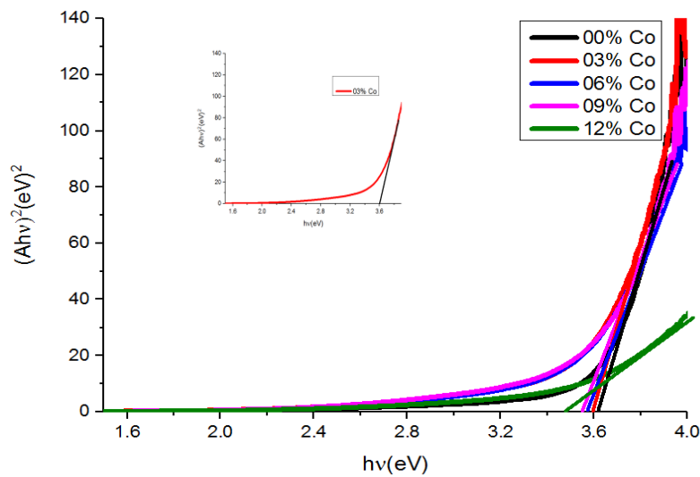
الشكل (17.III): منحنى تغيرات (Ah\nu)^2 بدلالة ( h\nu ) لأغشية أكسيد النيكل النقية والمطعمة.
