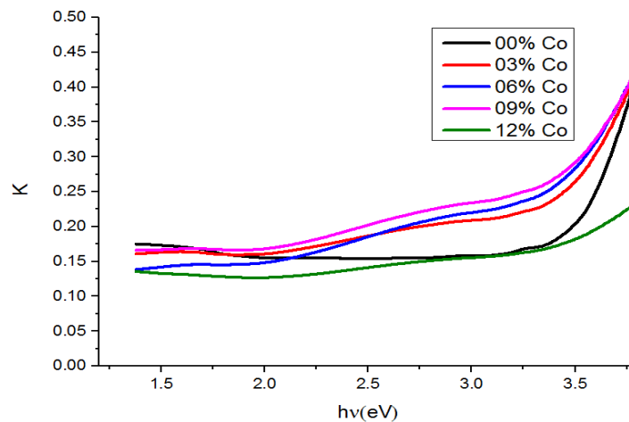
الشكل(20.III): معامل الخمود لأغشية أكسيد النيكل النقي والمطعم بالكوبالت.
