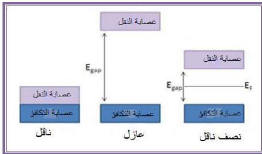
الشكل (1.I): مخطط حزم الطاقة للمواد الناقلة وأنصاف النواقل والعوازل [9].
