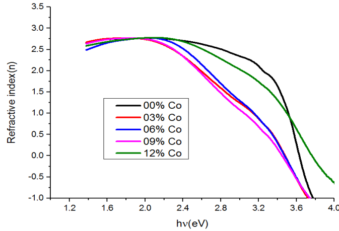
الشكل (21.III): معامل الإنكسار لأغشية أكسيد النيكل النقية والمطعمة بالكوبالت.
