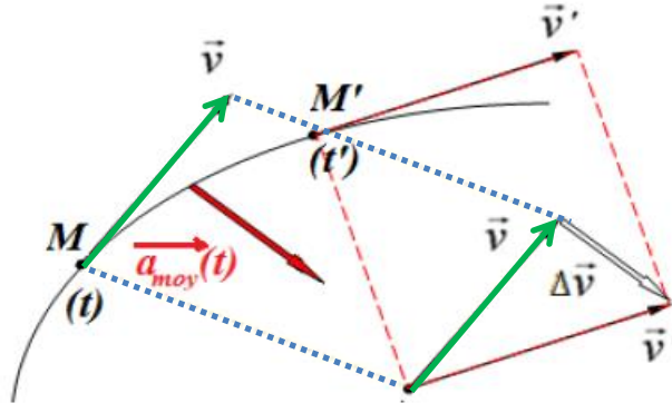
الشكل (4-I): شعاع التسارع المتوسط
