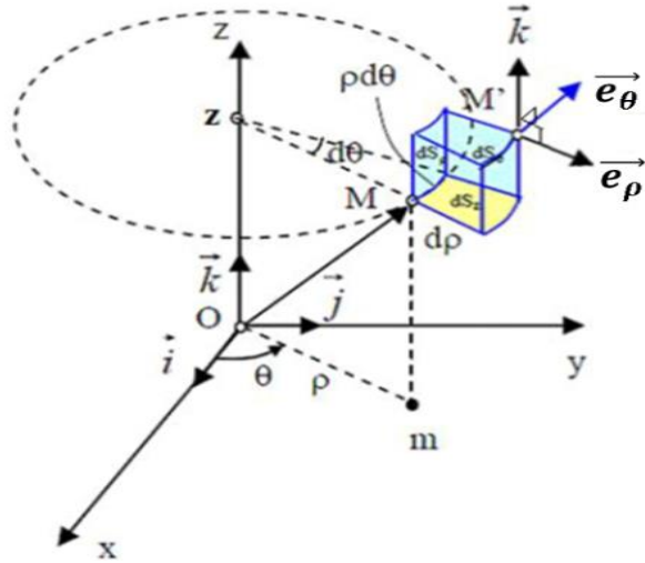
الشكل (I-18): الانتقال العنصري في المعلم الاسطواني
