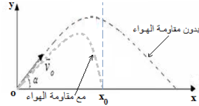
الشكل (12-I): تمثيل مسار قذيفة.
