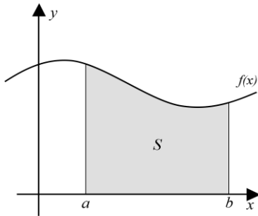
الشكل (1-1): مثال لحساب تكامل دالة
