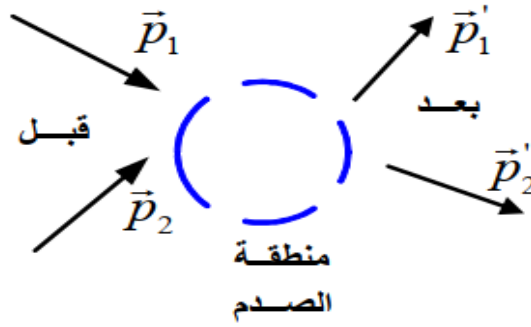
الشكل (5-I): تمثيل التصادم المرن
