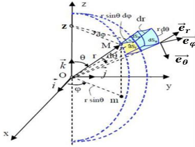
الشكل (I-19): الانتقال العنصري في المعلم الكارتيبي
