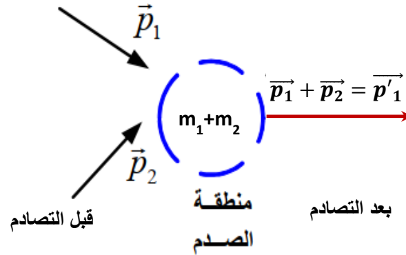
الشكل (6-I): تمثيل التصادم اللين
