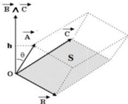
الشكل (II-11): الجداء الثلاثي المختلط
