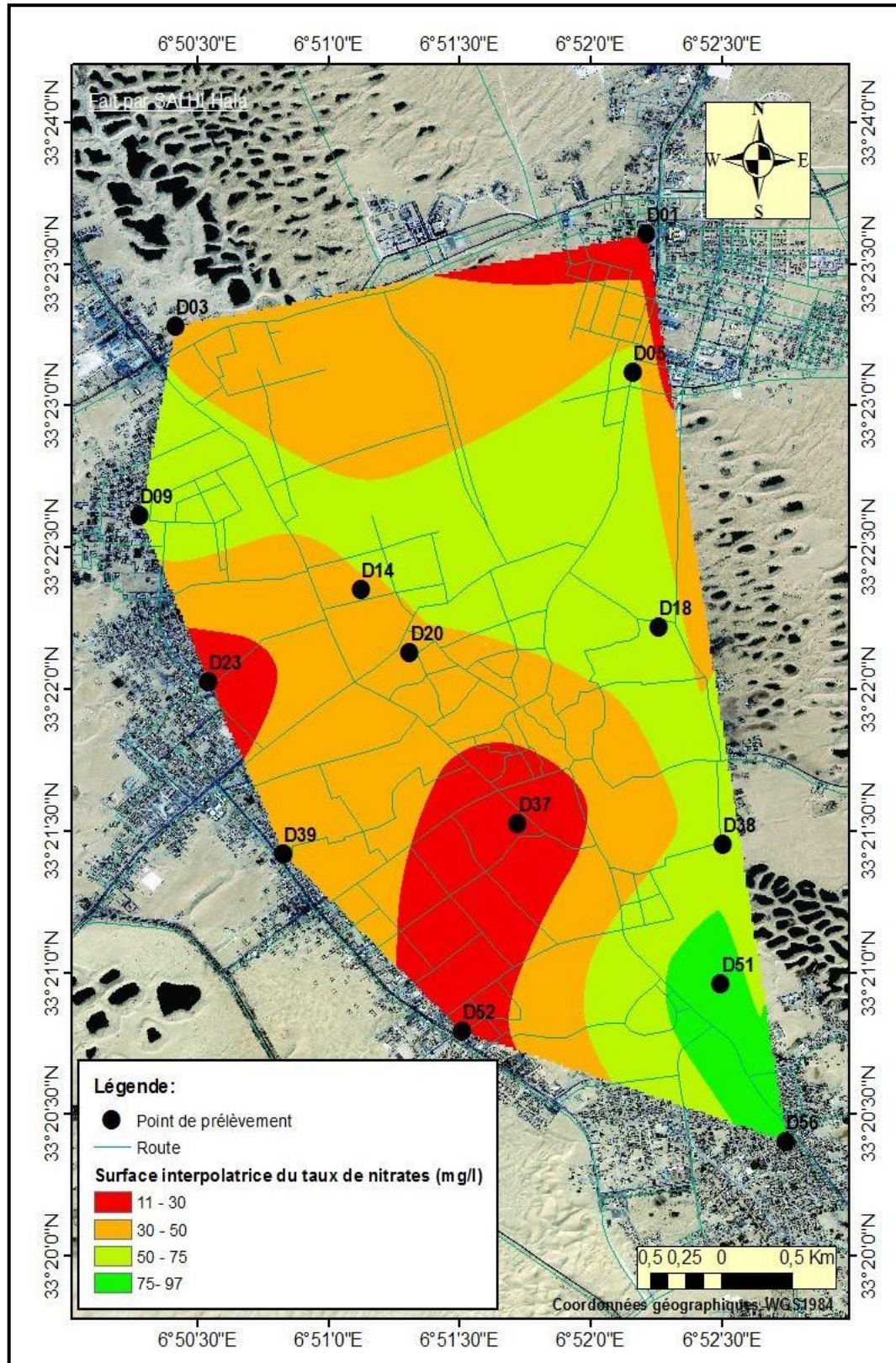
Figure (III.18) : Carte du Nitrates (2009) (Salhi H., 2016).
