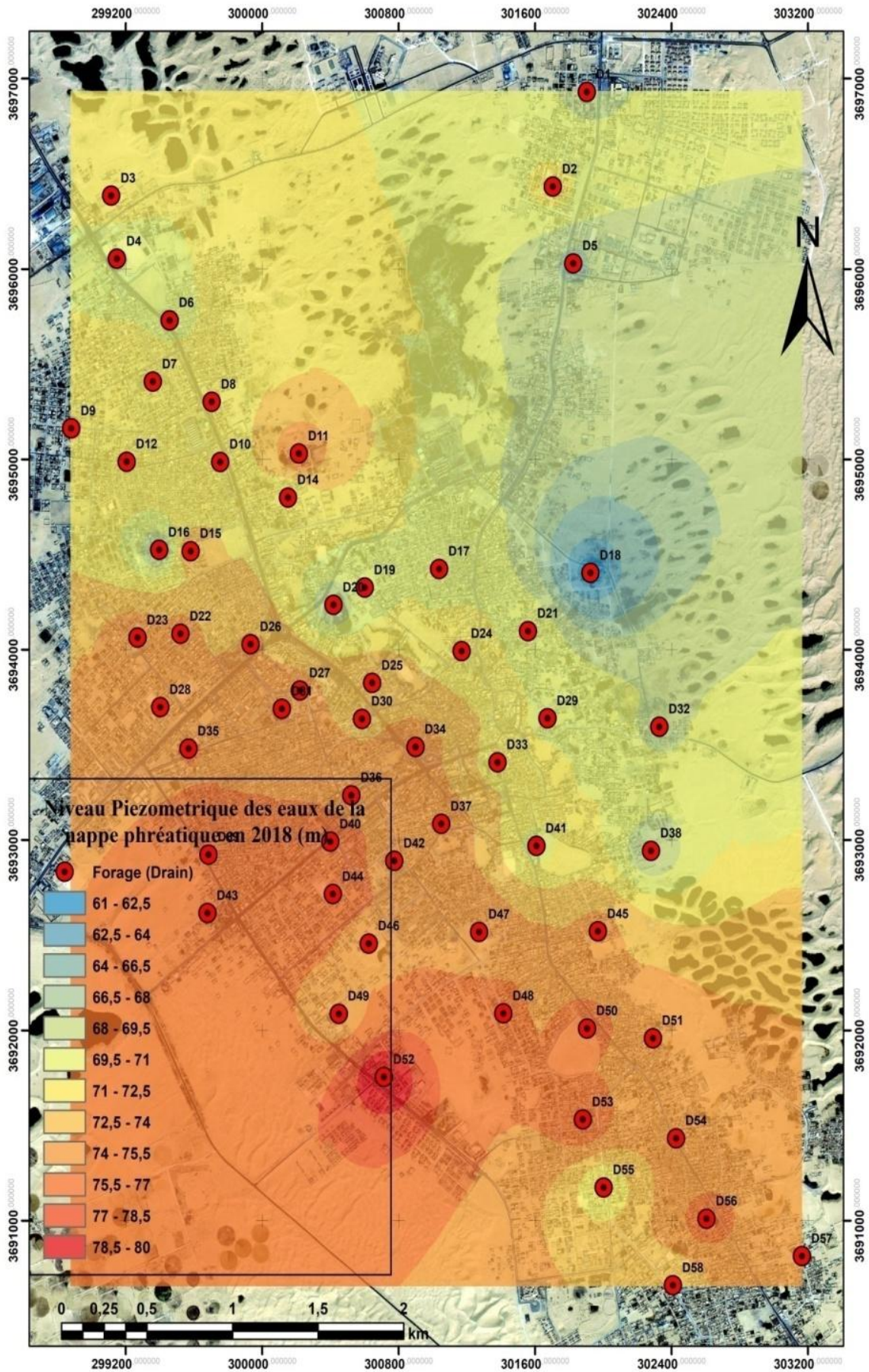
Figure (III.10) : Carte piézométrique de la nappe phréatique en 2018.
