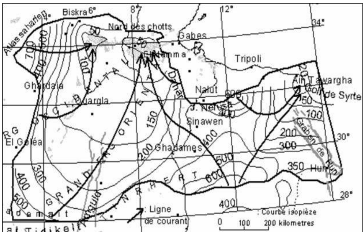
Figure (II.2): Limites de l'aquifère du Complexe terminale avec les niveaux piézométrique et les sens d'écoulement (Baba SY et al. 2006)
