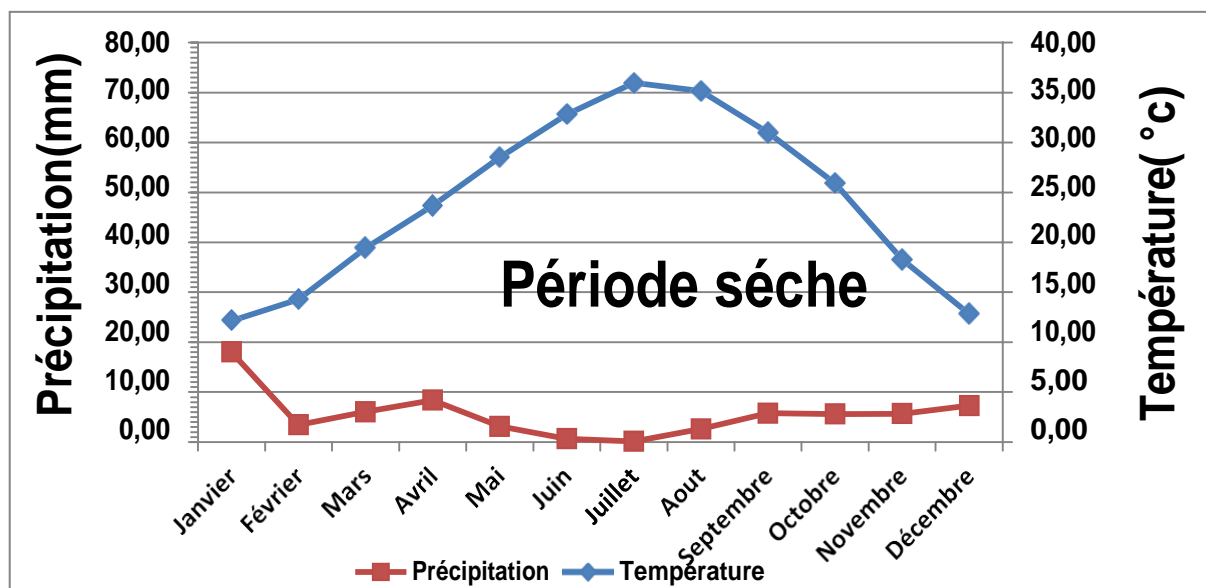
Figure (I.14): Diagramme Ombrothermique de la région d'Oued Souf (1990-2015).
