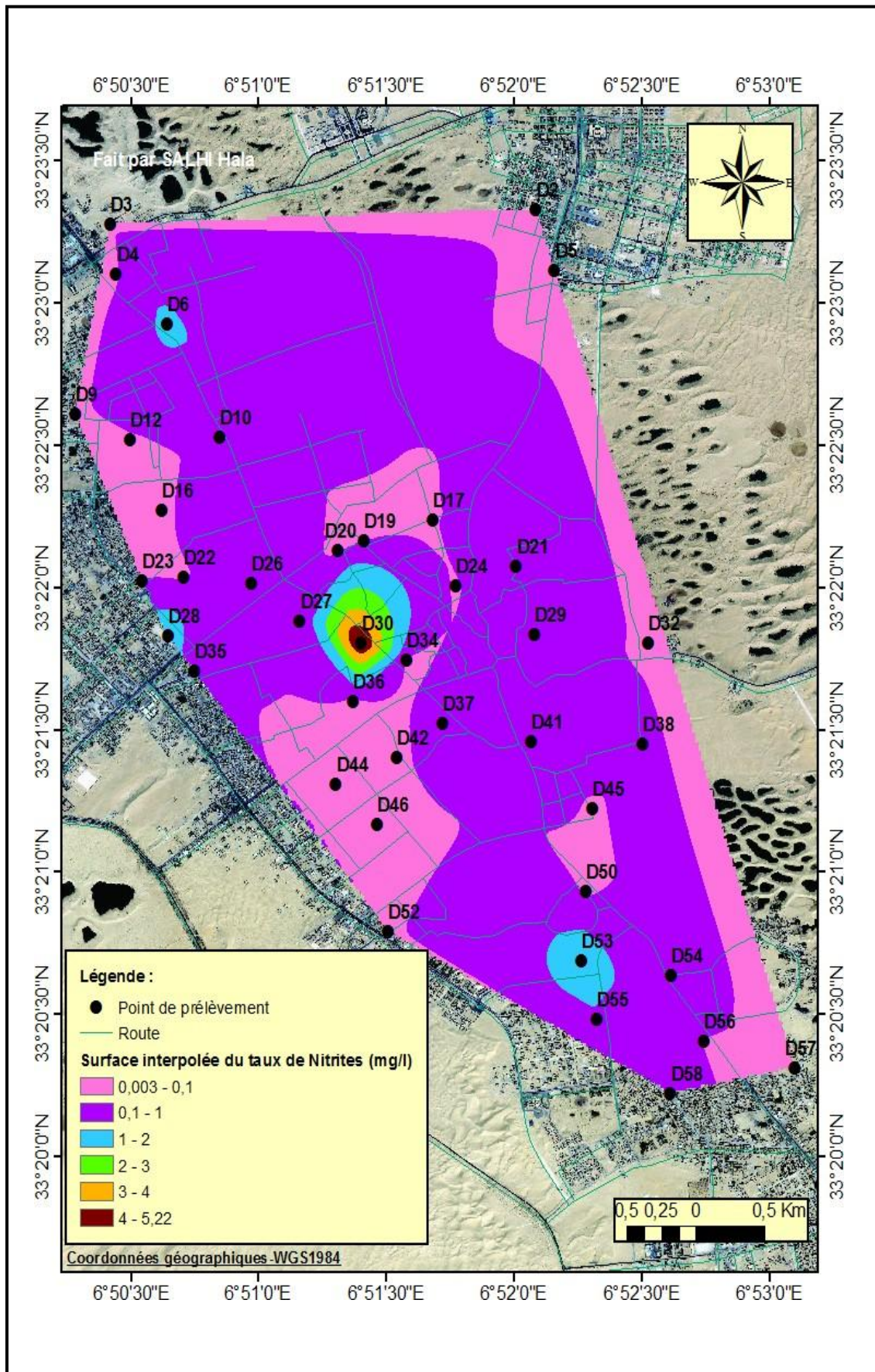
Figure (III.21) : Carte du Nitrites (Salhi H., 2016).
