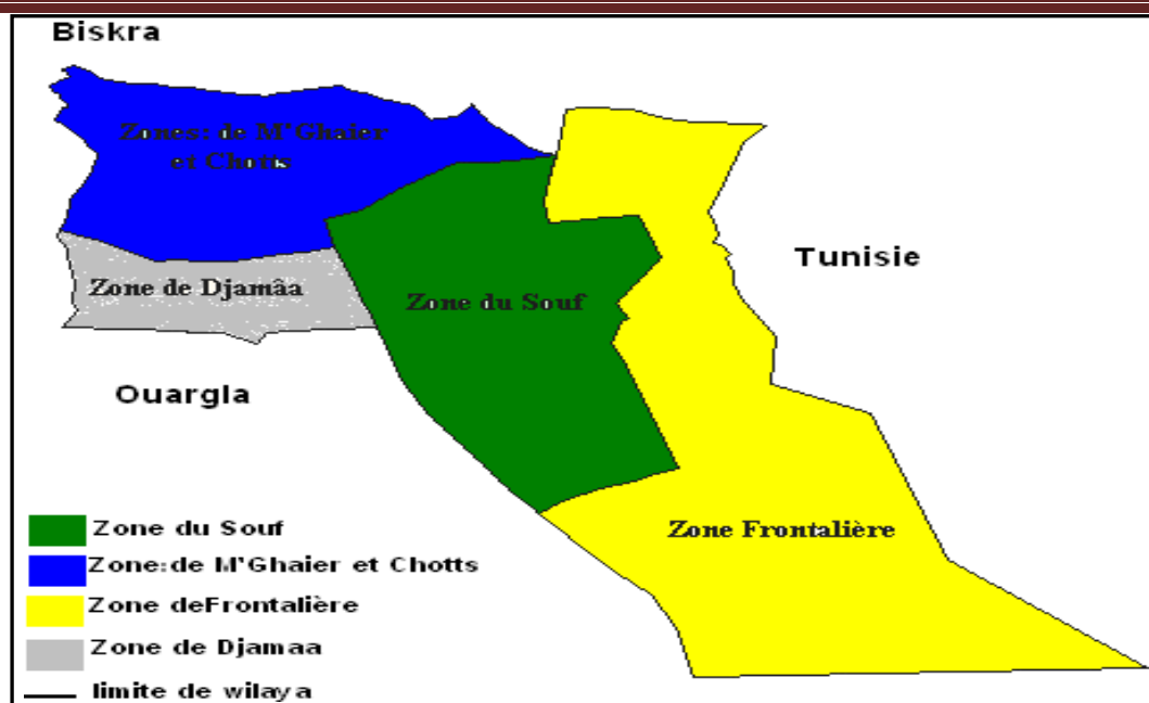
Figure (I.2) : Les Secteurs de la Wilaya d'El Oued. (ANRH 2005)
