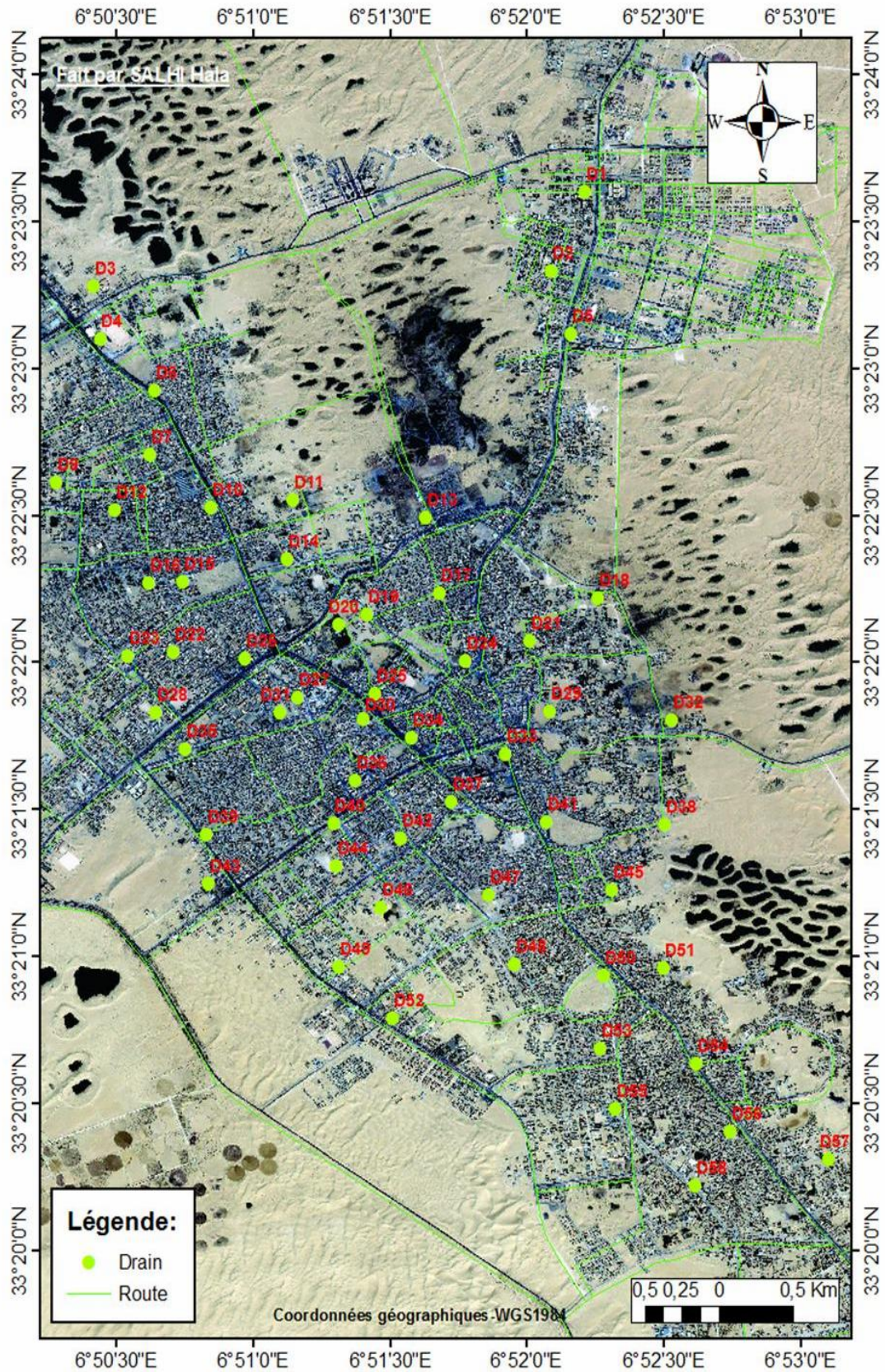
Figure(III.2): Localisation des 58 forages de réseau de drainage vertical (Salhi H., 2016).
