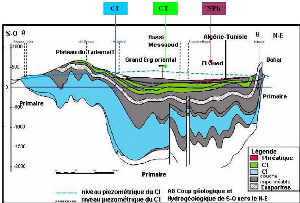
Figure (II.4) : Coupe hydrogéologique synthétique de Sahara Septentrionale (UNESCO, 1972)
