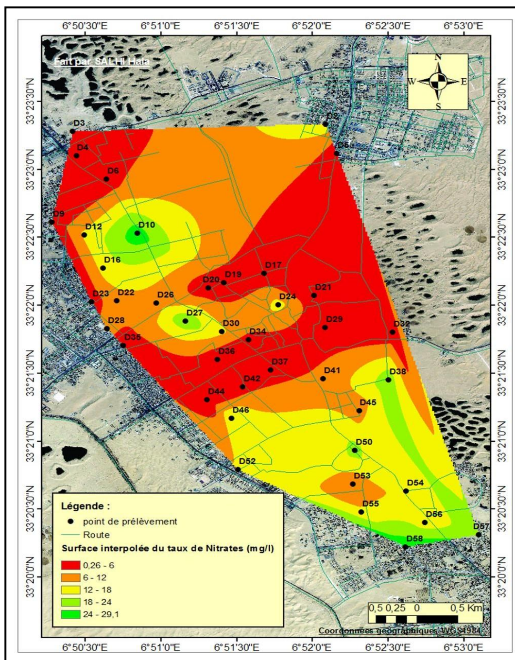
Figure (III.19) : Carte du Nitrates (Salhi H., 2016).
