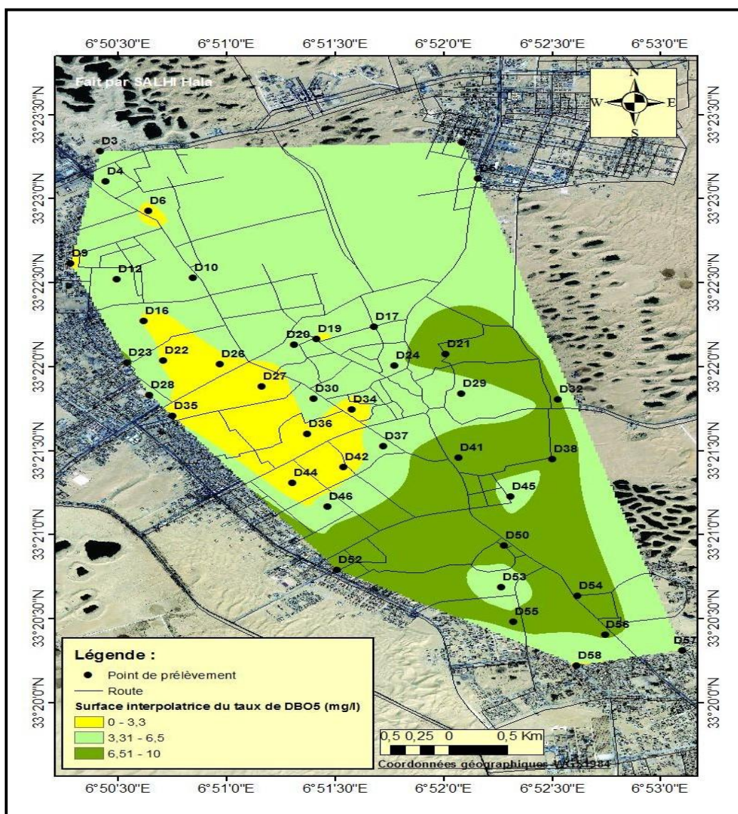
Figure (III.23) : Carte de Demande Biologique en Oxygène à 5 jours (Salhi H., 2016).
