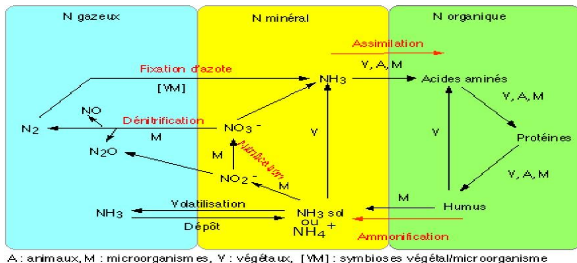
Figure (III.17) : Cycle de l'azote.(Derouiche ;2014)
