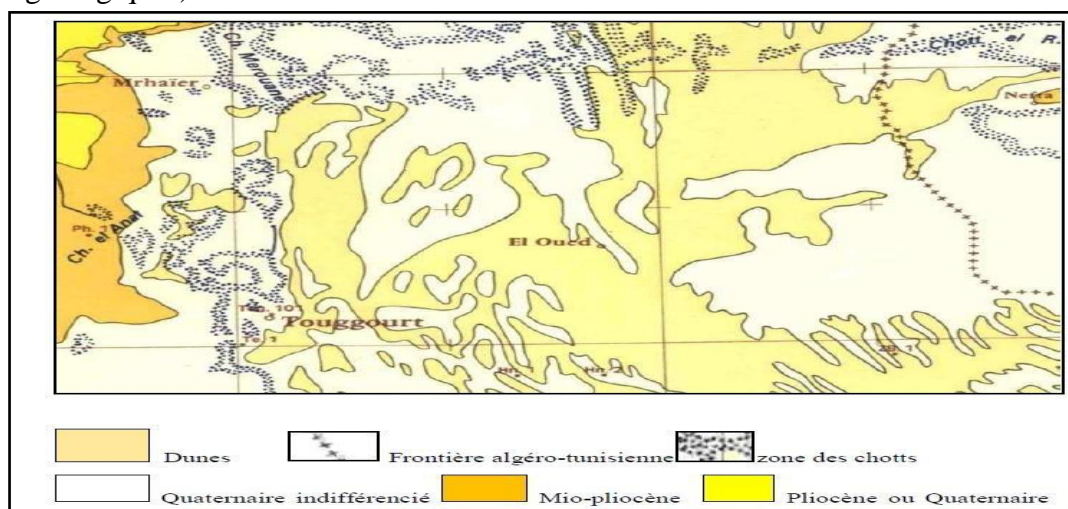
Figure(I.4): Carte géologique de la région d'El-Oued (extrait de la carte du Sahara septentrional) (Bisson, 1971)
