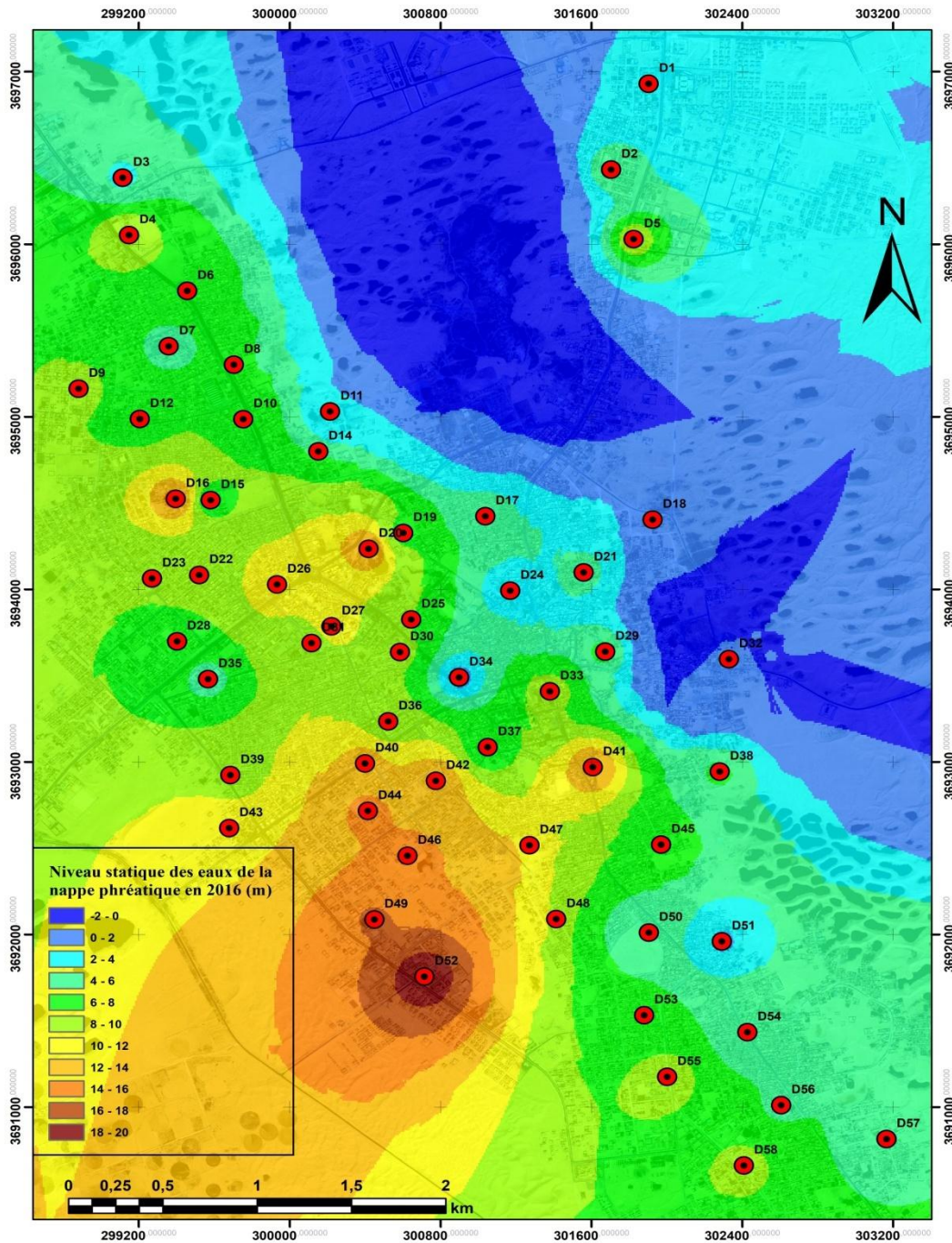
Figure (III.8) : Carte de niveau Statique des eaux de la nappe phréatique en 2016.
