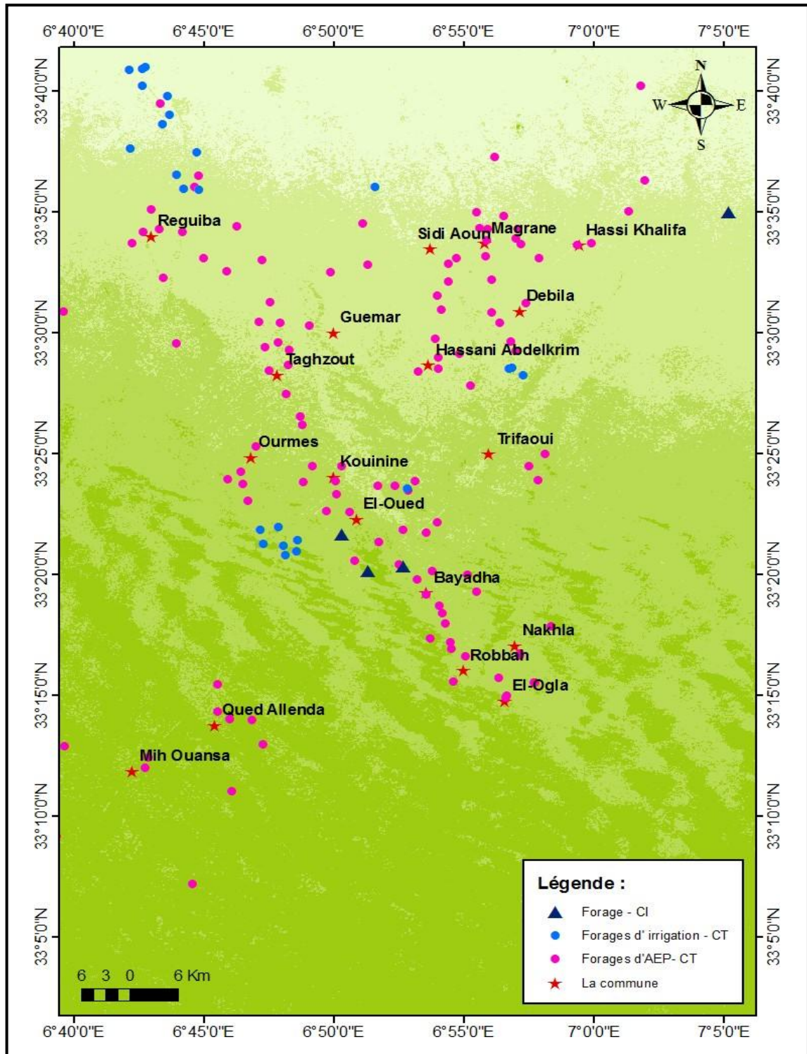
Figure (II.7) : Carte d'inventaire des Forages du CT et CI sur la vallée d'Oued-Souf (2015)
