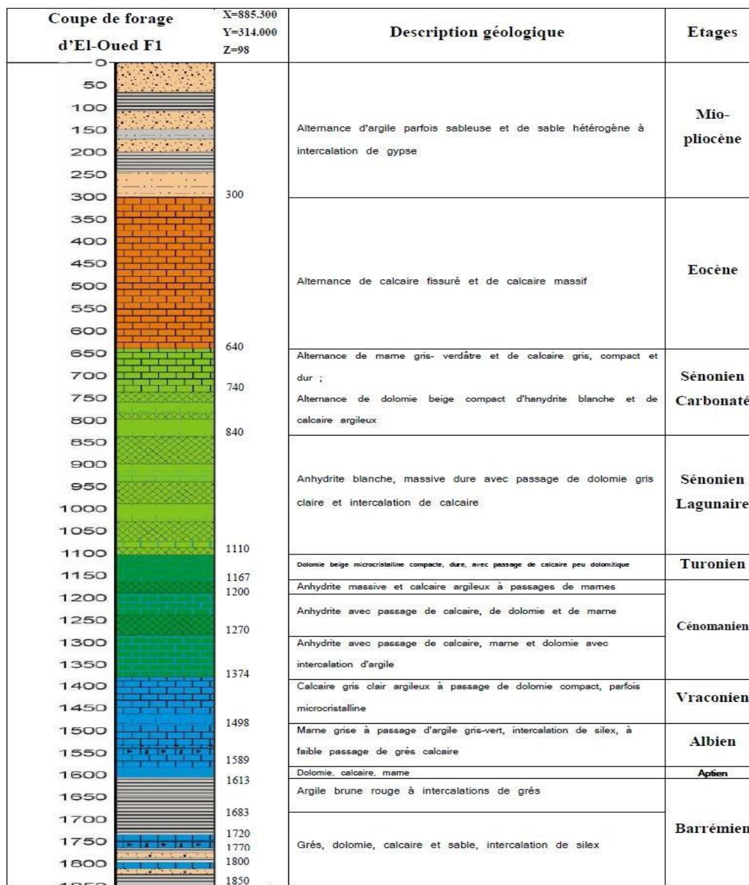
Figure. (I.3) : La lithostratigraphie du forage F1, (ANRH, 1993)
