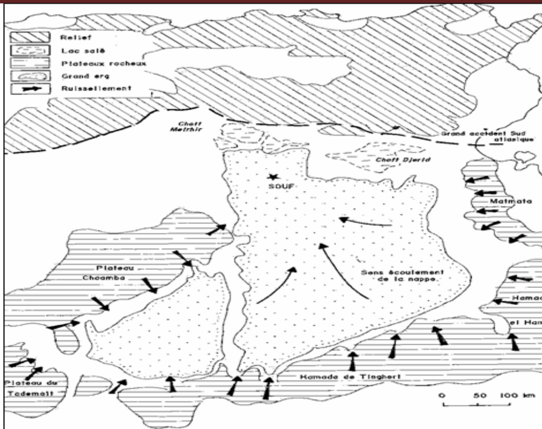
Figure (II.1): Zone d'alimentation de la nappe phréatique et le sens d'écoulement (Cote Marc, 2006)
