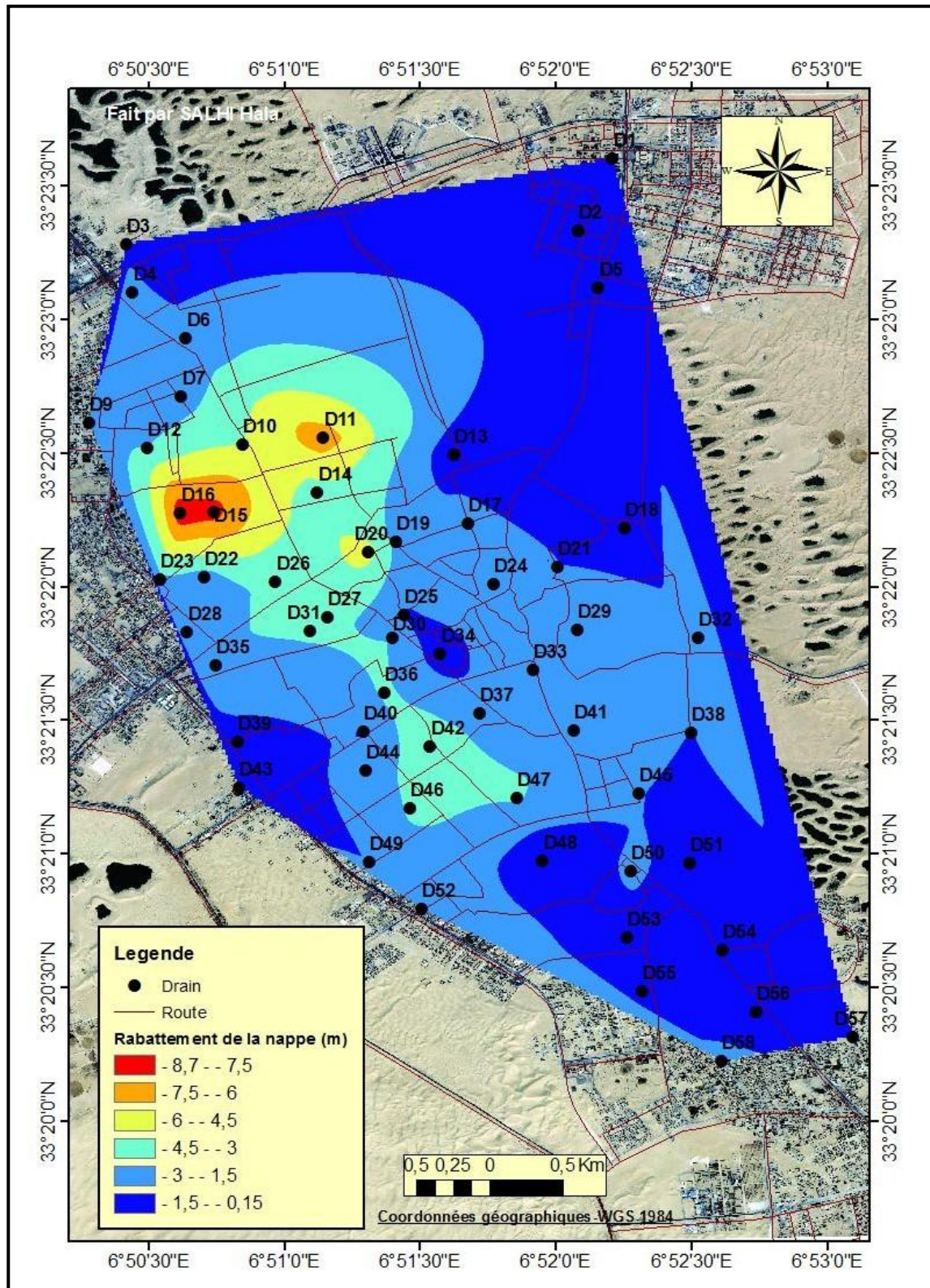
Figure (III.6) : Carte d'évolution du niveau piézométrique entre l'année 2008 et l'année 2014 de la ville d'El-Oued(Salhi H., 2016).
