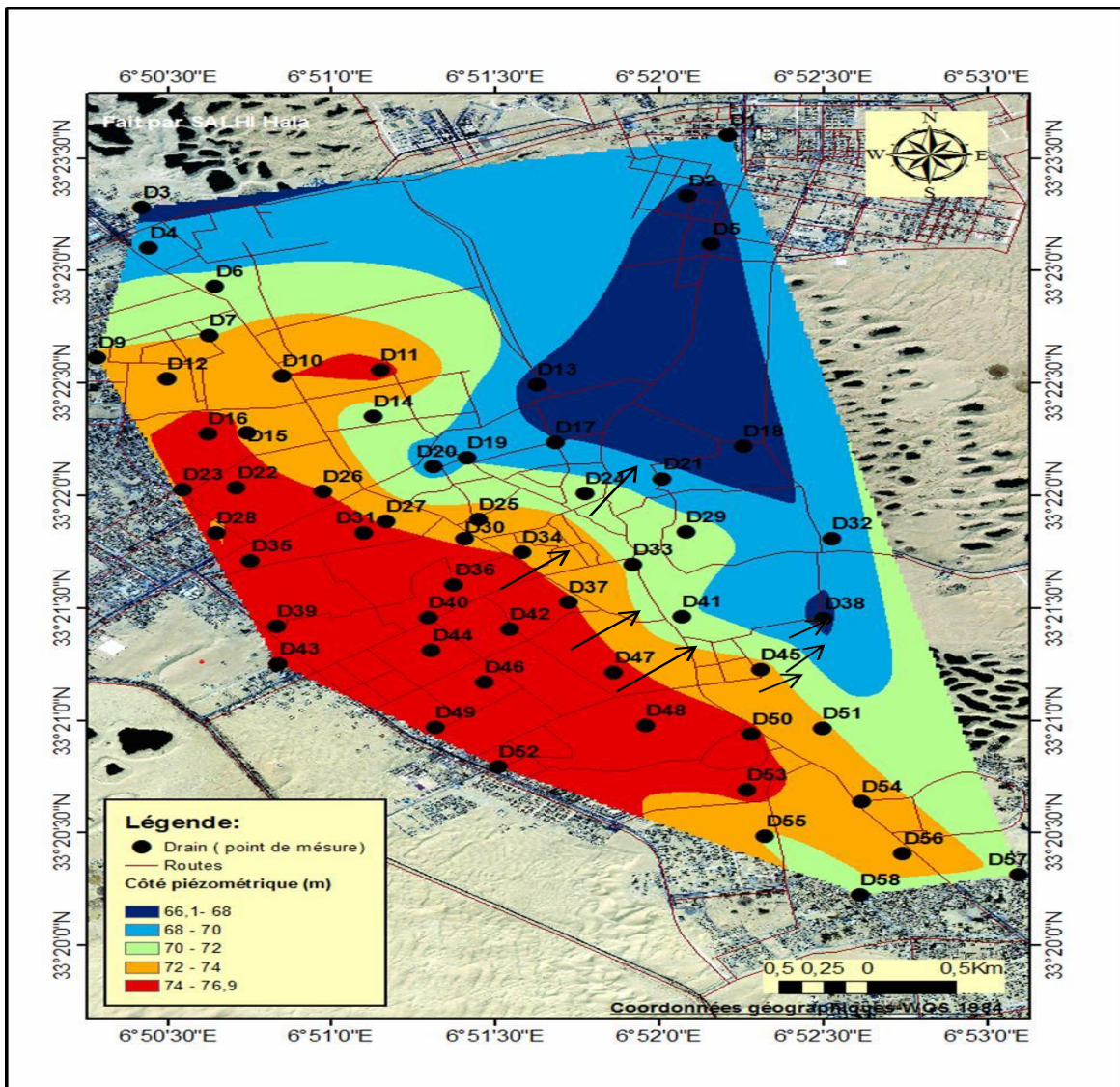
Figure (III.4) : Carte piézométrique de la nappe phréatique à l'année 2008 (Salhi H., 2016).
