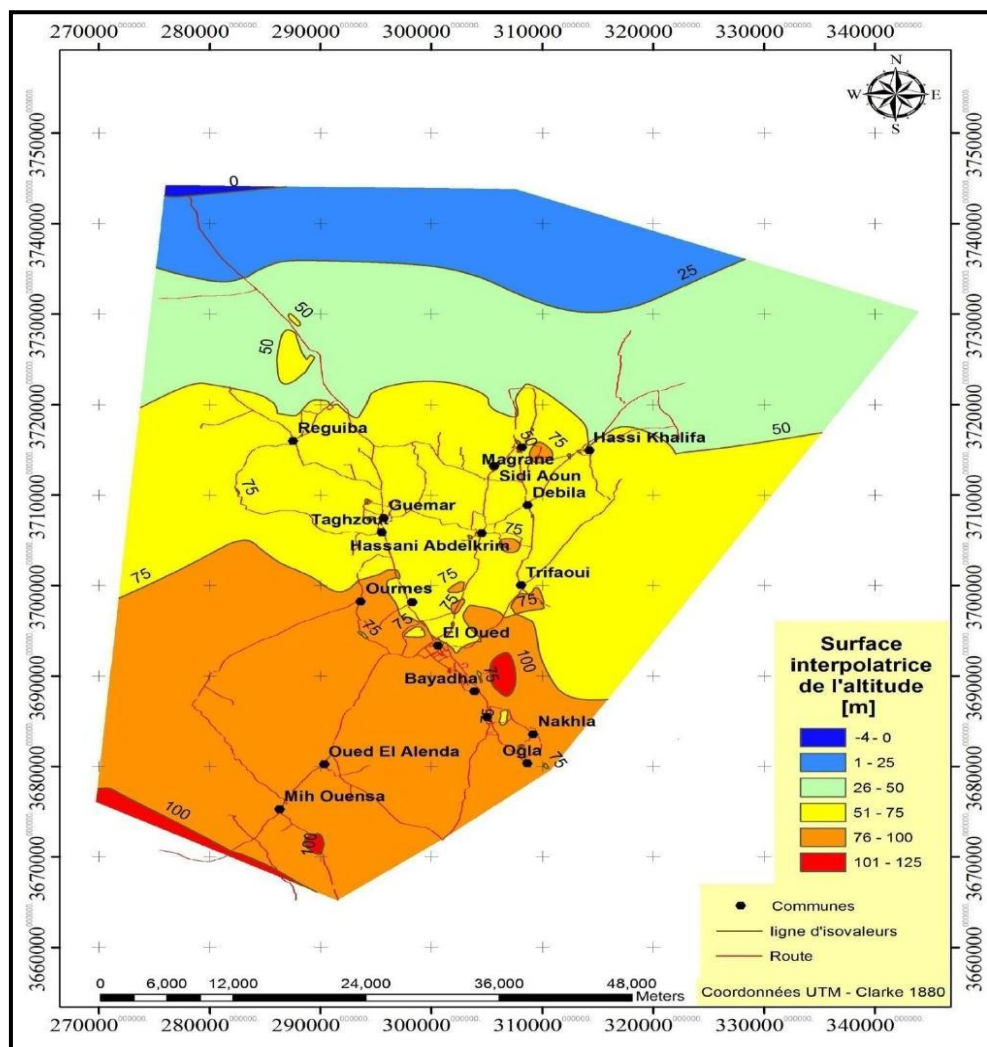
Figure (I.5) : Carte topographique de la région de souf
