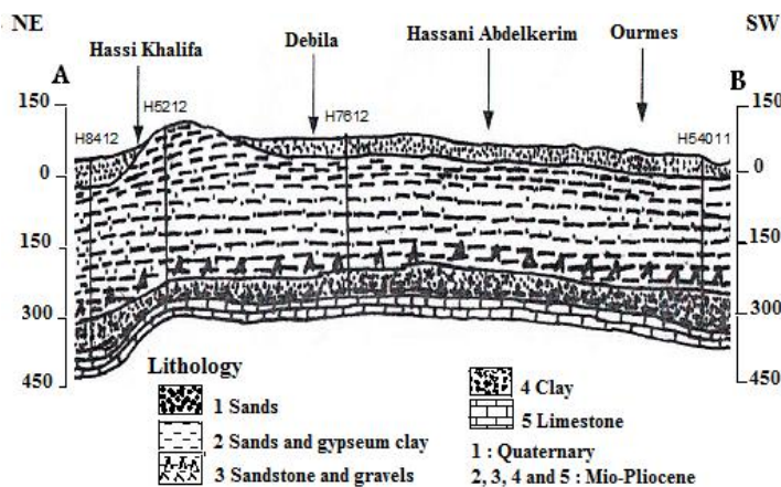
Fig 1. Coupe géologique extraite par les logs de forages profonds
