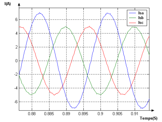
FigureIII.12.Variation des courants.
