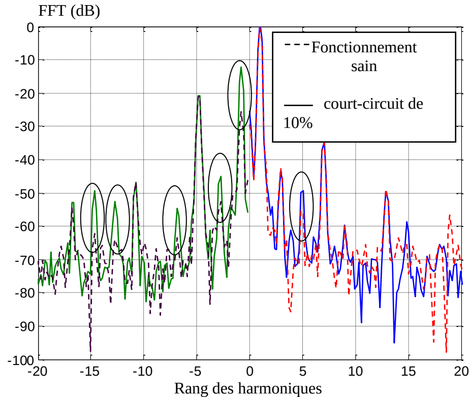
Figure III.20. Spectre fréquentiel du vecteur de Park des courants statoriques expérimentaux
