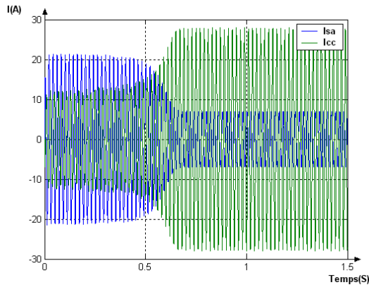
FigureIII.11.Variation des courants.
