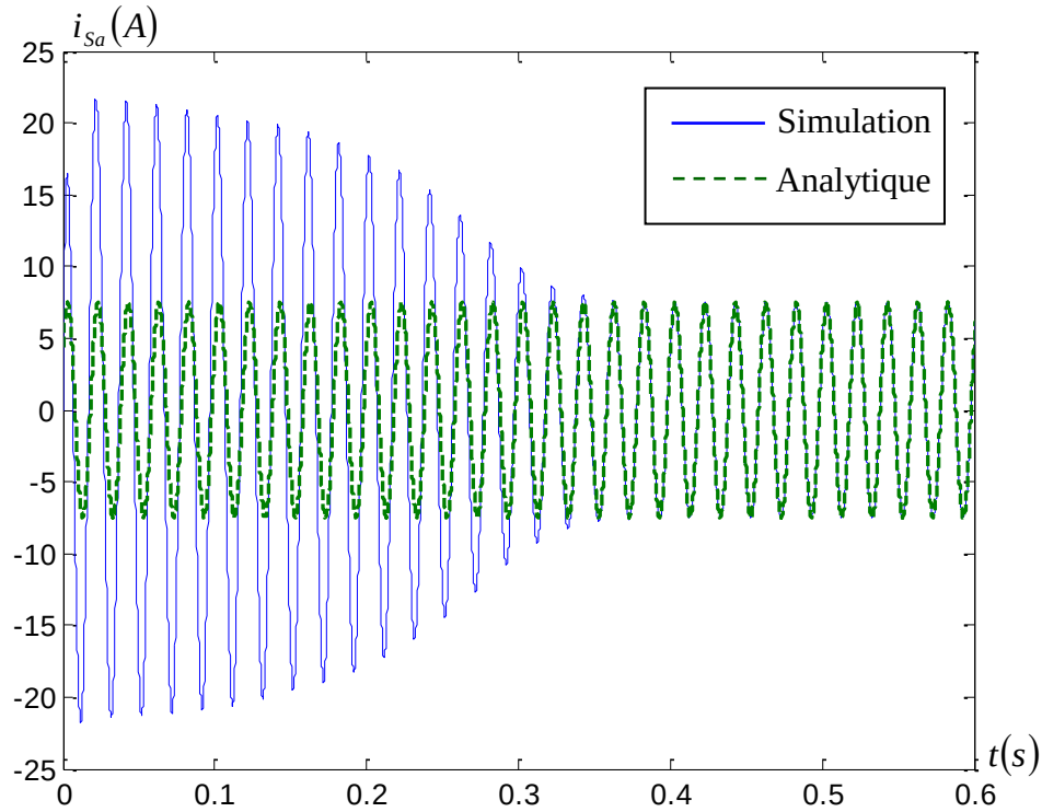
Figure III.18. Courant statorique de la phase a.
