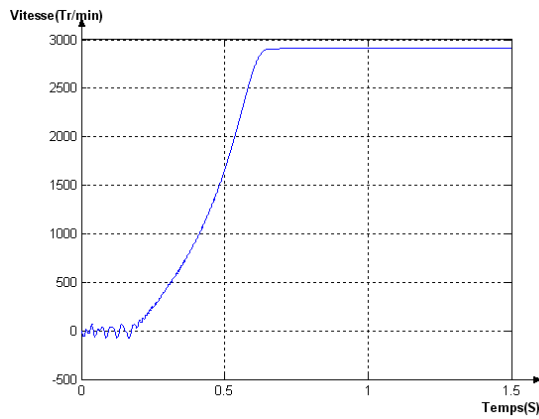
FigureIII.13.Variation de la vitesse
