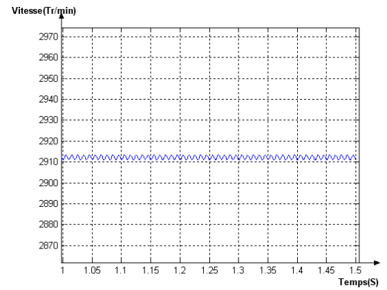
FigureIII.14.Variation de la vitesse
