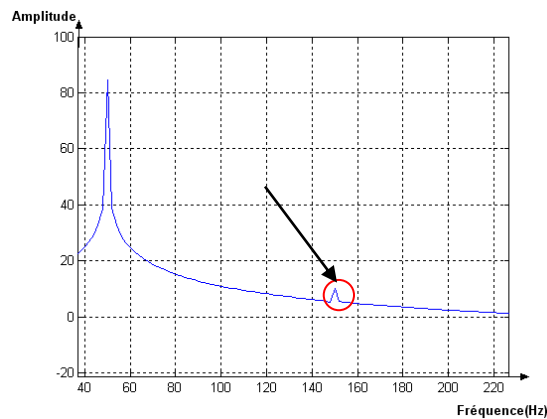
Figure III.17. Zoom du spectre du courant statorique.
