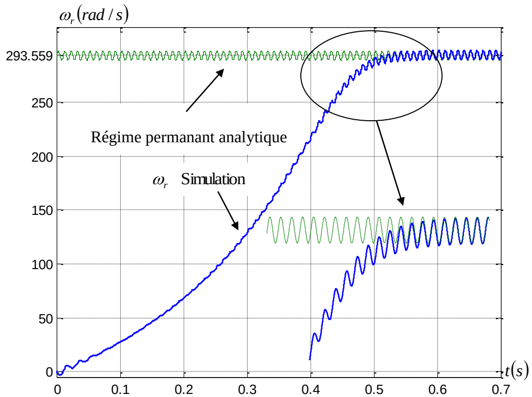
Figure 4.19. Vitesse en présence d'un défaut de 50%.
