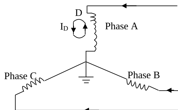
FigureIII.1. Configuration des enroulements statoriques avec un court-circuit dans la phase « a ».
