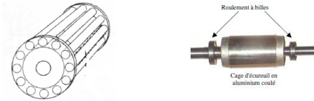
Figure I.3. Le rotor à cage d'écureuil.
