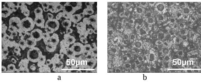
Figure 1. Microstructure de la fonte FB ; a : à l'état brut de coulée, b : à l'état traité
