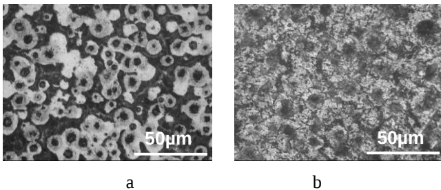
Figure 3. Microstructure de la fonte B; a : à l'état brut de coulée, b : à l'état traité
