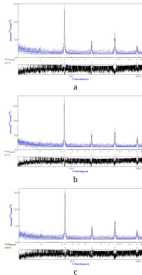
Figure 5. Spectre de diffraction X. a : fonte de base (FB), b : fonte alliée (A), c : fonte (B)
