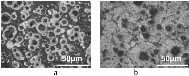
Figure 2. Microstructure de la fonte A; a : à l'état brut de coulée, b : à l'état traité
