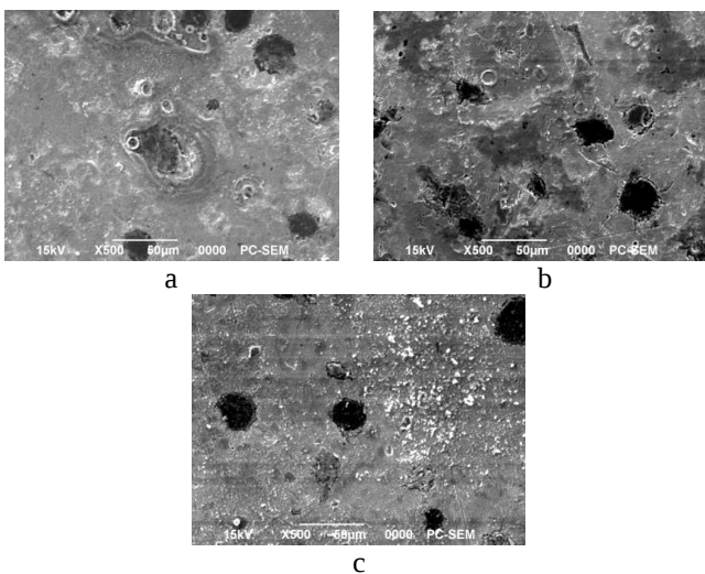
Figure 4. Microstructure (MEB) à l'état traité ; a : fonte de base FB, b : fonte A, c : fonte B
