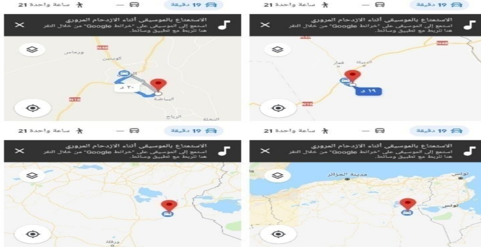
صورة توضح موقع الجمعية بالتفصيل
