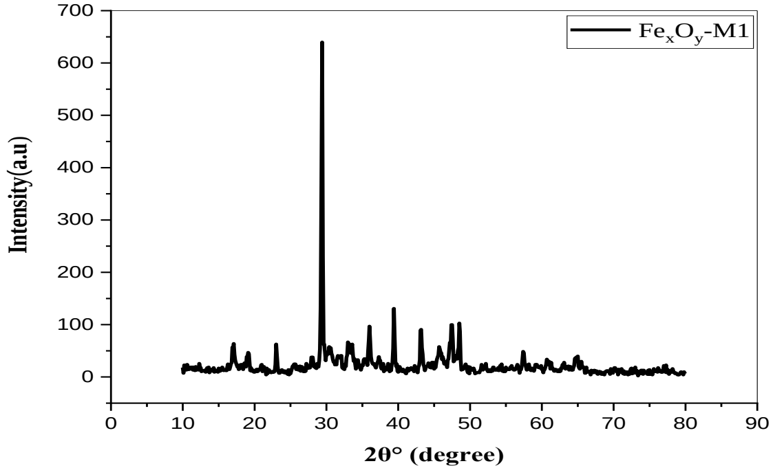
الشكل (16.IV): نمط حيود الأشعة السينية لعينة \text{Fe}_x\text{O}_y\text{-M1} .
