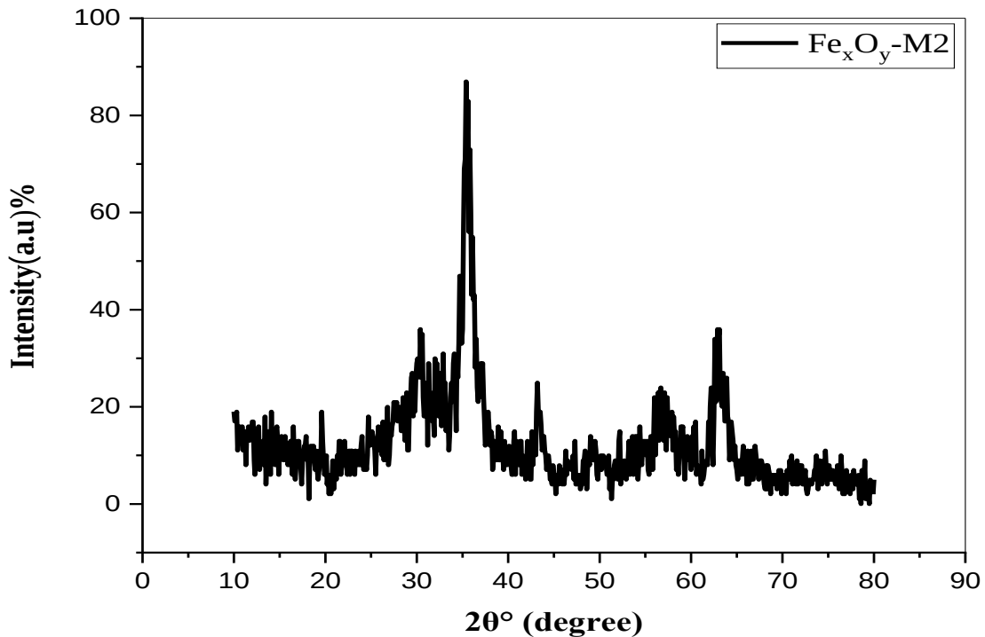
الشكل (III. 18): نمط حيود الاشعة السينية لعينة Fe x O y -M2.
