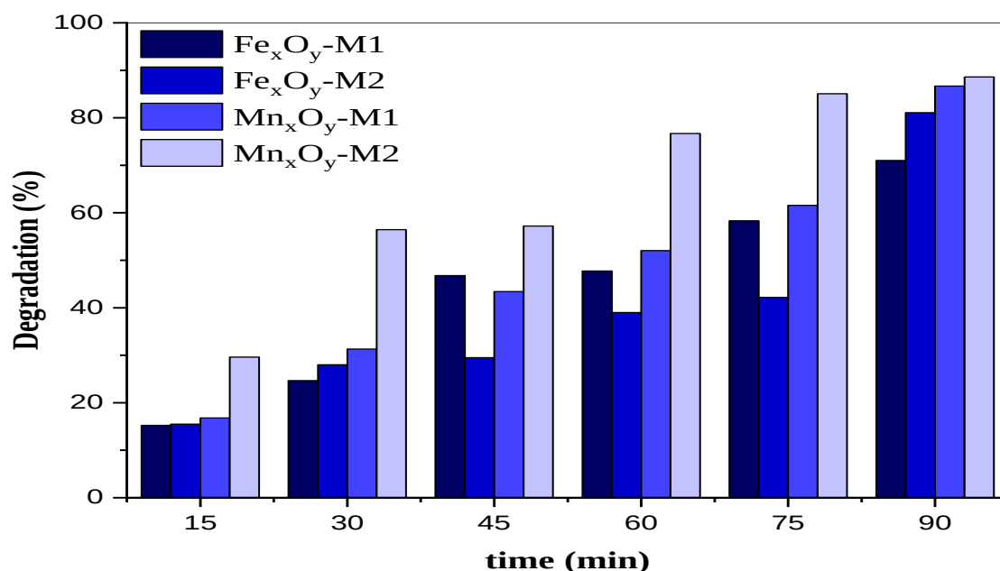
الشكل (23.IV): تطور كفاءة إزالة صبغة أزرق الميثيلين باستعمال العينات Fe x O y -M1 ، Fe x O y -M2 ، Mn x O y -M1 و Mn x O y -M2 مع زمن التشعيع.
