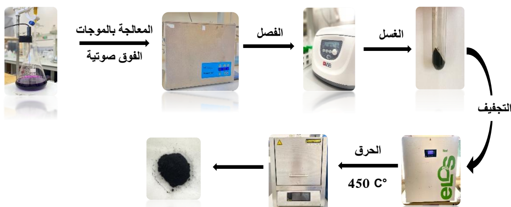
الشكل (11.III): التصنيع الأخضر لجسيمات أكسيد المنغنيز بطريقة المستخلص النباتي لأوراق الزيتون.
