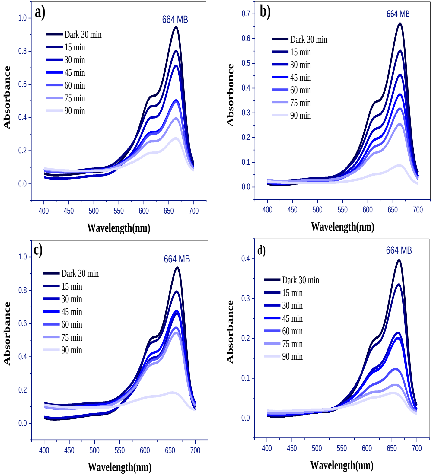
الشكل (22.IV): أطياف الأشعة فوق البنفسجية-المرئية (UV-Vis) لصبغة أزرق الميثيلين تحت التشعيع الشمسي باستعمال المحفزات (a) \text{Fe}_x\text{O}_y\text{-M1} ، و (b) \text{Mn}_x\text{O}_y\text{-M1} ، و (c) \text{Fe}_x\text{O}_y\text{-M2} ، و (d) \text{Mn}_x\text{O}_y\text{-M2} .
