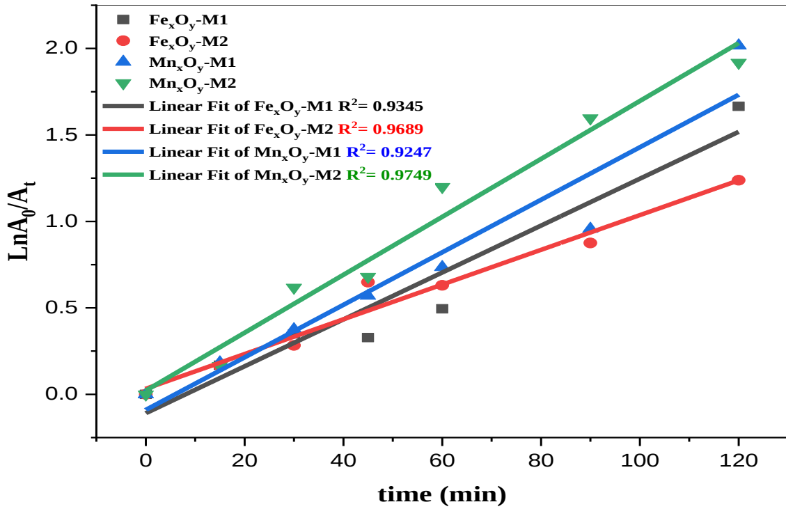
الشكل (27.IV): منحنيات نموذج الرتبة الأولى (PFO) للعينات Fe x O y -M2، Fe x O y -M1، Mn x O y -M1 و Mn x O y -M2.
