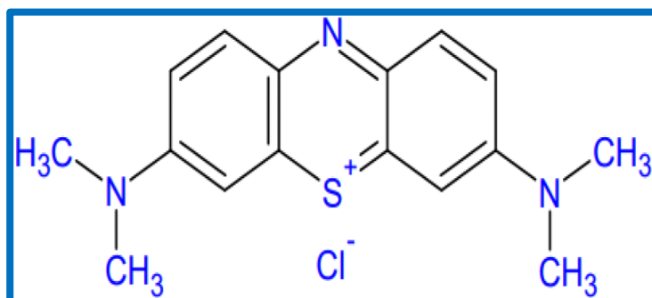
الشكل (12.III): البنية الجزيئية لصبغة أزرق الميثيلين.
