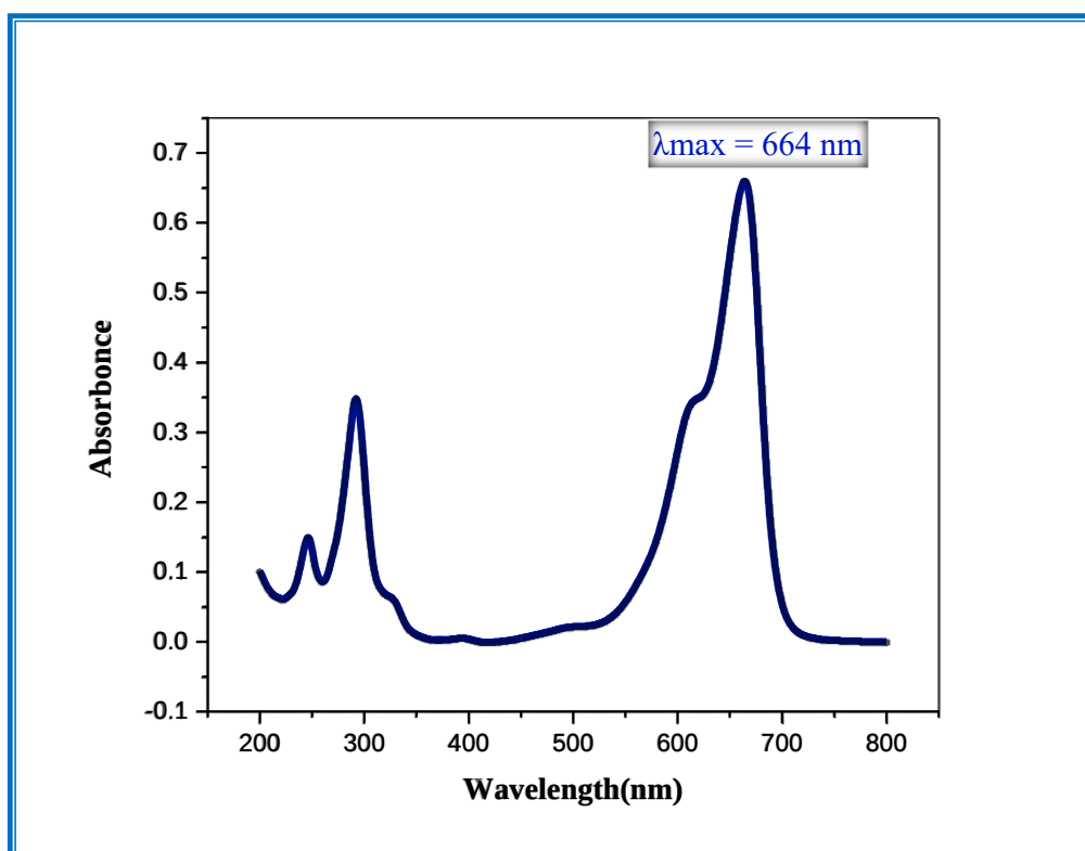
الشكل(13.III): منحنى الطول الموجي الأعظمي لصبغة أزرق الميثيلين.
