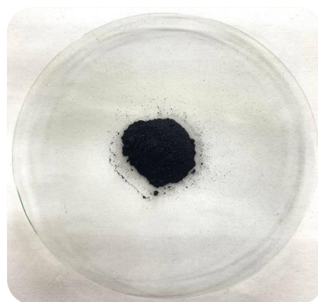
\text{Mn}_3\text{O}_4\text{-M2}
