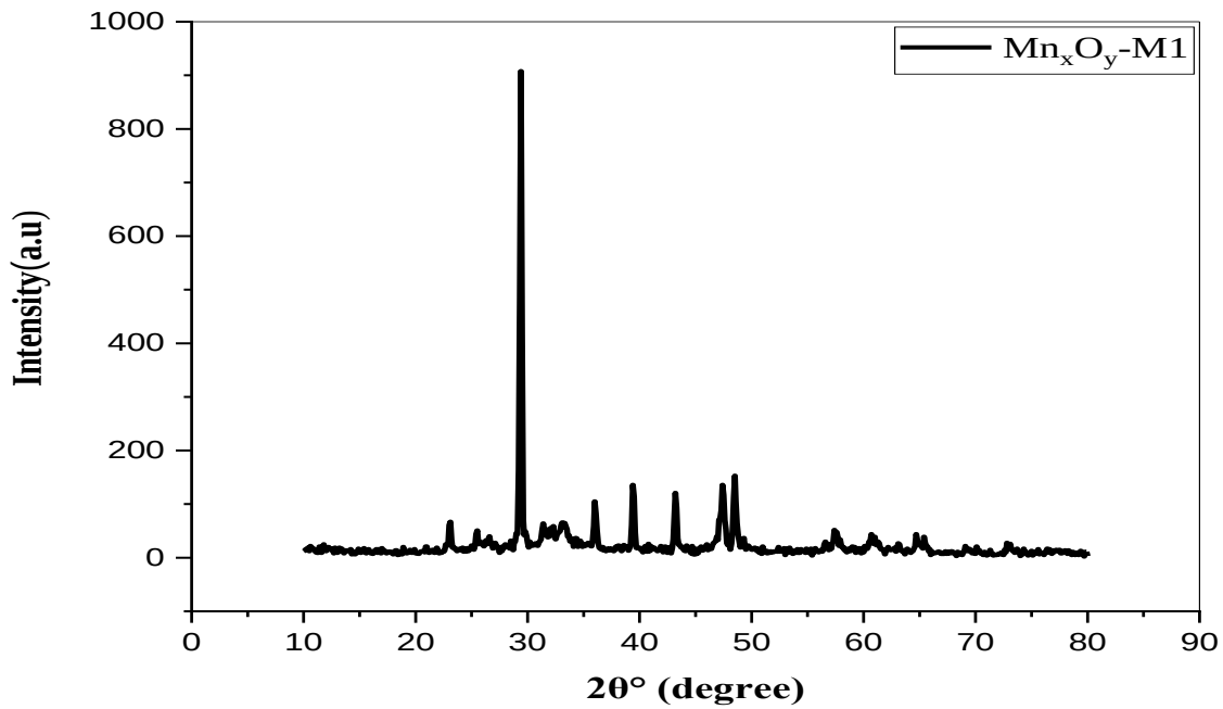
الشكل (17.III): نمط حيود الأشعة السينية لعينة \text{Mn}_x\text{O}_y\text{-M1} .
