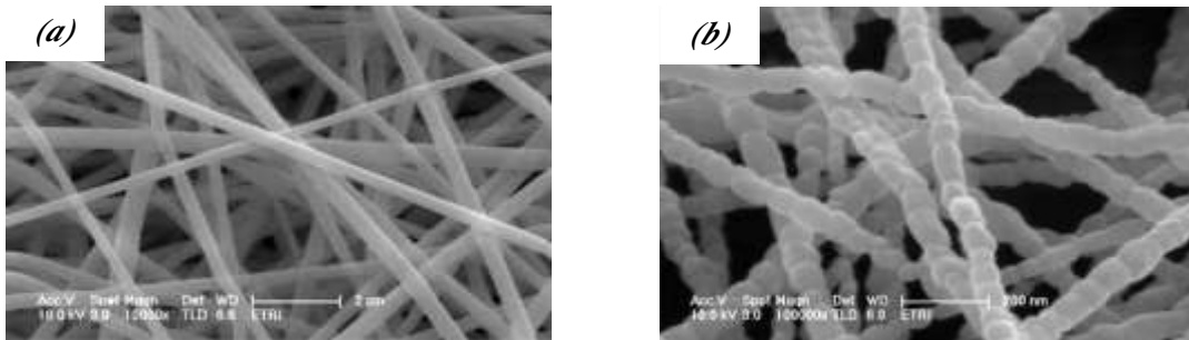
Figure II.5 : Images MEB : (a) fibres d'acétate de PVA / composites de zinc, (b) fibres après calcination à 700°C (J. Park et al ; 2009)
