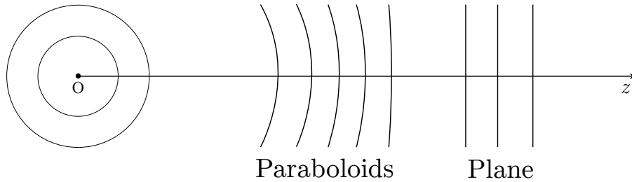
Fig. 1.12: Paraxial Helmholtz
